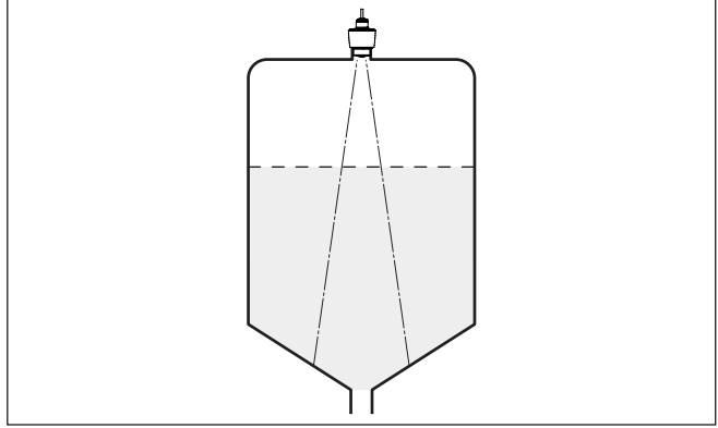
Res. 7: Radar sensörünün konik tabanlı haznelere montajı
