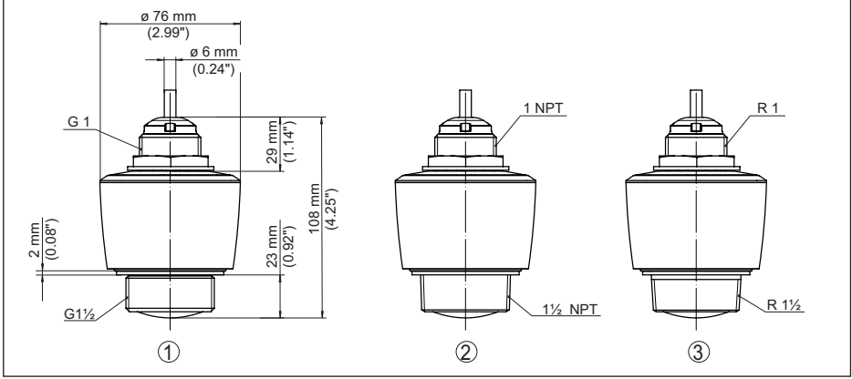
Res. 28: Ebatlar - VEGAPULS C 11
