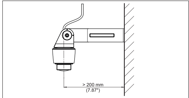
Res. 4: Bir montaj dirseği ile montaj
