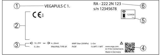
Res. 2: Model etiketinin yapısı (Örnek)
