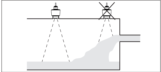
Res. 9: İçeri akan dolun malzemesinde radar sensörünün montajı
