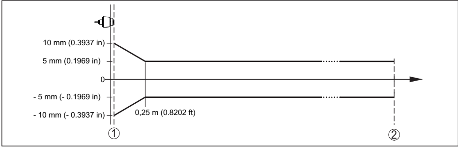
Res. 27: Referans koşullarına tabi ölçüm sapması 10)
