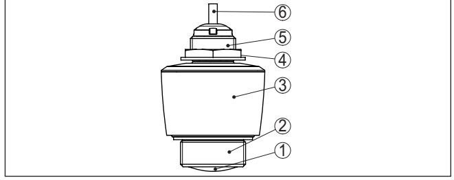
Res. 1: VEGAPULS C 11 cihazının öğeleri
