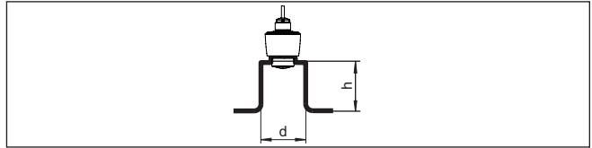
Res. 11: Boru soketleri ebatları standarttan farklı olduğunda
