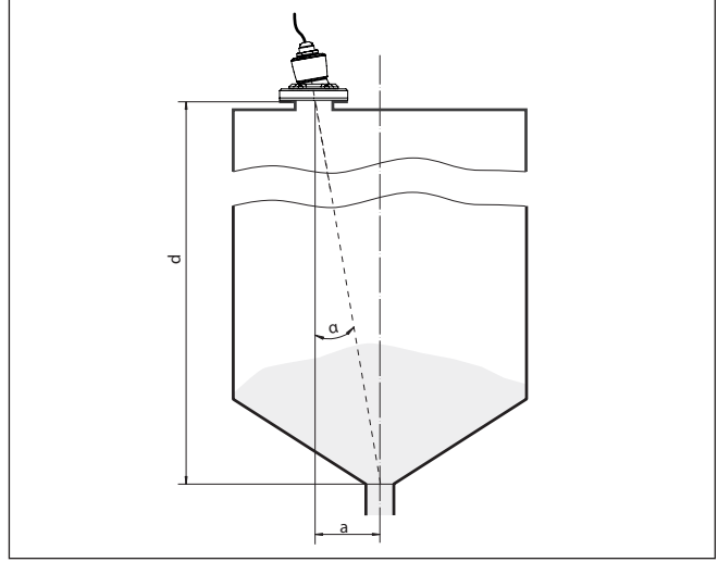
Res. 15: VEGAPULS C 11 hizalamaya göre kurulum için öneri
