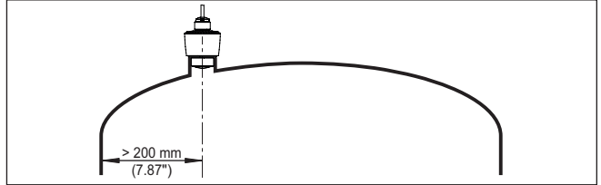
Res. 6: Radar sensörünün yuvarlak hazne tavanlarına montajı
