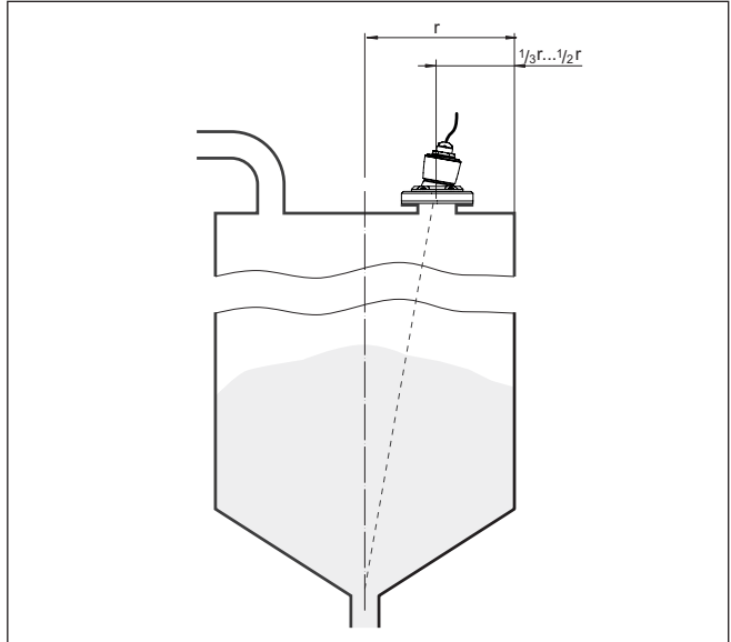
Res. 14: Montaj konumu ve ayar
