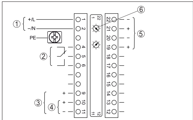
Fig. 13: Elektronica- en aansluitruimte bij niet-Ex instrumenten en instrumenten met niet-intrinsiekveilige stroomuitgang
