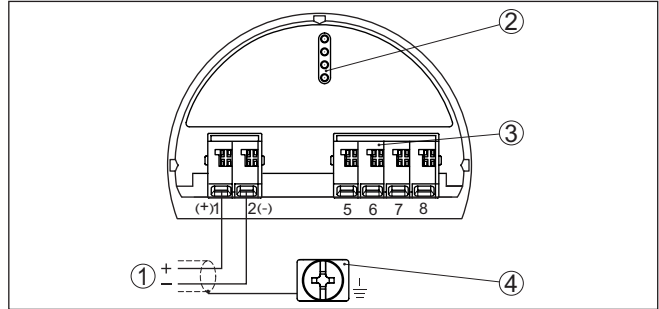
Abb. 16: Bedien- und Anschlussraum (Ex ia) bei Geräten mit eigenem Stromausgang
