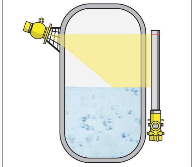
Res. 4: Bir tanktaki dolum ölçümü
