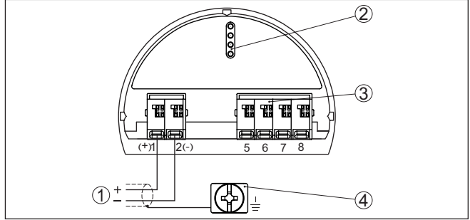
Res. 16: Bünyesinde güvenli olan sinyal çıkışlı cihazlarda kumanda ve bağlantı bölümü (Ex ia)
