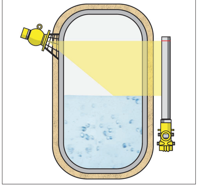
Res. 7: Isı yalıtımlı, ısıtılmış bir haznede dolun seviyesinin ölçümü
