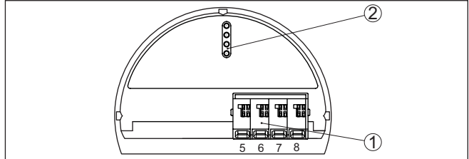
Res. 10: Ex olmayan cihazlar ve bünyesinde güvenliği olmayan akım çıkışlı cihazlarda kumanda ve bağlantı bölmesi
