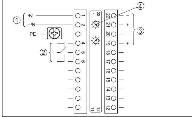
Res. 15: Bünyesinde güvenliği olan akım çıkışlı cihazlarda elektronik bölme ve bağlantı bölgesi (Ex d)
