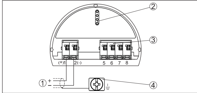
Res. 16: Bünyesinde güvenliği olan akım çıkışlı cihazlarda kumanda ve bağlantı bölgesi (Ex ia)
