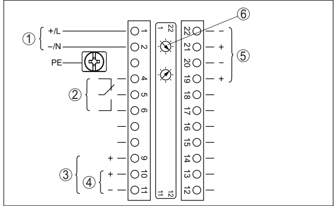
Res. 13: Ex olmayan cihazlar ve bünyesinde güvenliği olmayan akım çıkışlı cihazlarda elektronik bölme ve bağlantı bölümü
