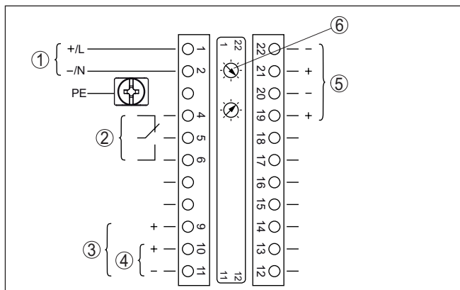
Fig. 9: Compartimento do sistema eletrônico e de conexão - em aparelhos Não-Ex e aparelhos com saída de corrente sem segurança intrínseca.
