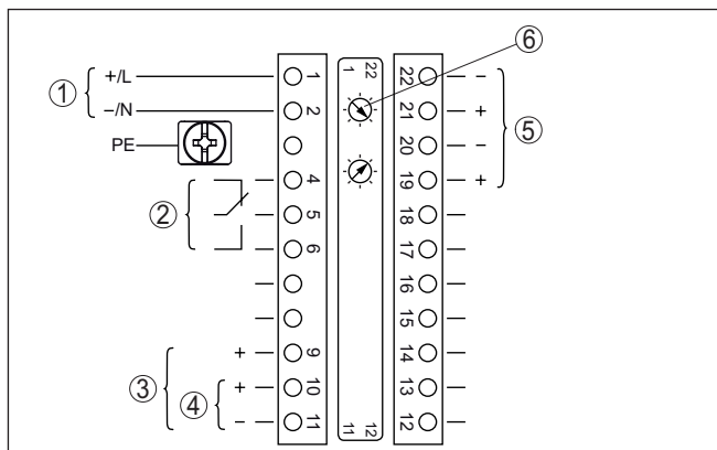
Fig. 13: Compartimento do sistema eletrônico e de conexão - em aparelhos Não-Ex e aparelhos com saída de corrente sem segurança intrínseca.
