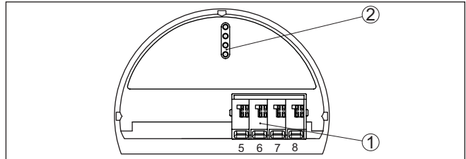
Res. 10: Ex olmayan cihazlar ve bünyesinde güvenliği olmayan akım çıkışlı cihazlarda kumanda ve bağlantı bölümü
