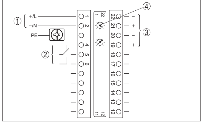
Res. 15: Bünyesinde güvenliği olan akım çıkışlı cihazlarda elektronik bölme ve bağlantı bölümü (Ex d)
