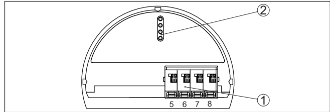
Res. 14: Ex olmayan cihazlar ve bünyesinde güvenliği olmayan sinyal çıkışlı cihazlarda kumanda ve bağlantı bölümü
