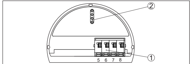
Res. 14: Ex olmayan cihazlar ve bünyesinde güvenliği olmayan sinyal çıkışlı cihazlarda kumanda ve bağlantı bölmesi
