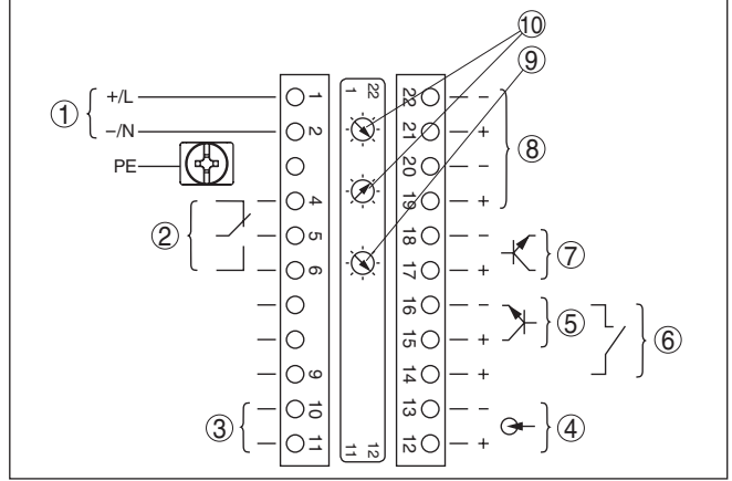
Res. 9: Ex olmayan cihazlar ve bünyesinde güvenliği olmayan sinyal çıkışı cihazlarda elektronik bölme ve bağlantı bölümü
