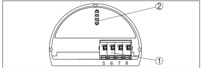
Res. 10: Ex olmayan cihazlar ve bünyesinde güvenliği olmayan sinyal çıkışı cihazlarda kumanda ve bağlantı bölümü
