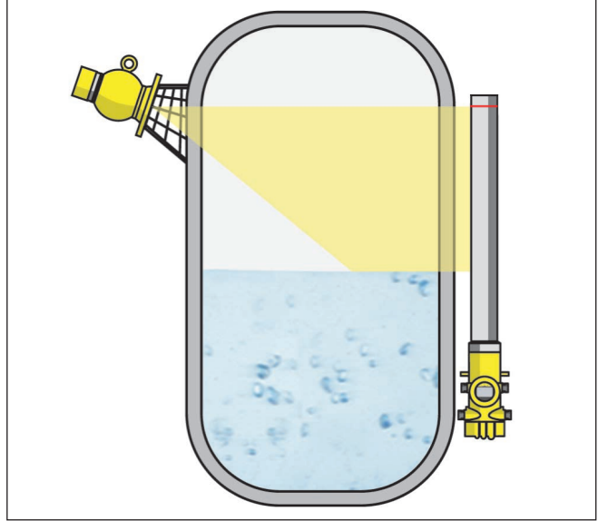
Res. 4: Bir tanktaki dolum ölçümü
