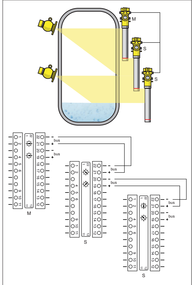
Res. 17: Birden fazla cihazın kademelenmesinde elektronik ve bağlantı bölmesi.
