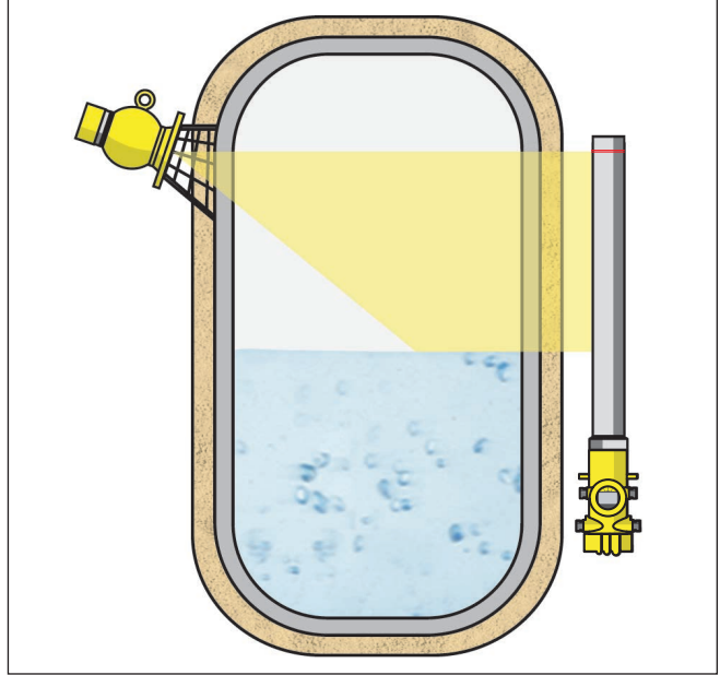
Res. 7: Isı yalıtımlı, ısıtılmış bir haznede dolum seviyesinin ölçümü
