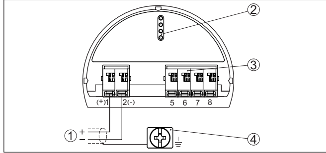
Res. 16: Bünyesinde güvenliğin akım çıkışı cihazlarda kumanda ve bağlantı bölmesi (Ex ia)
