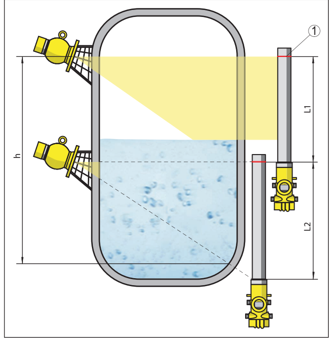
Res. 6: Takma pozisyonu - Kademeli düzen
