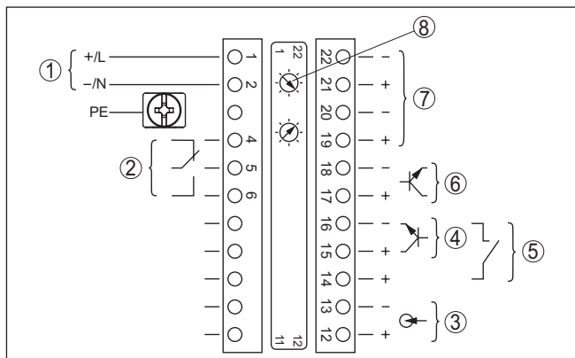
Rys. 15: Komora układu elektronicznego i przyłączy (Ex d) w przypadku przyrządów z iskrobezpiecznym wyjściem prądowym
