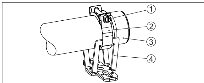
Fig. 6: Abrazadera de montaje
