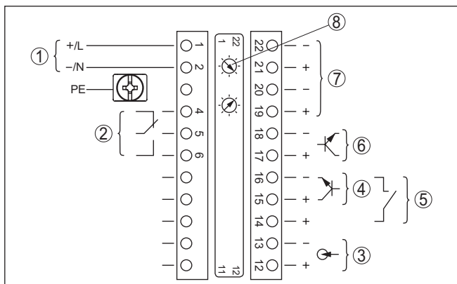
Figura 13: Vano dell'elettronica e di connessione (Ex d) per apparecchi con uscita in corrente a sicurezza intrinseca
