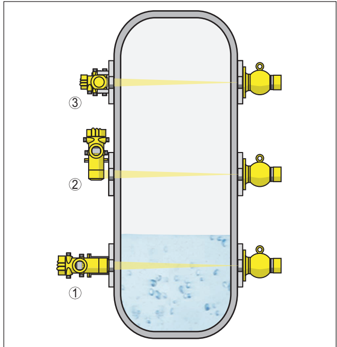
Figura 5: Posizione di montaggio - rilevamento di soglia di livello - esecuzione senza tubo rivelatore
