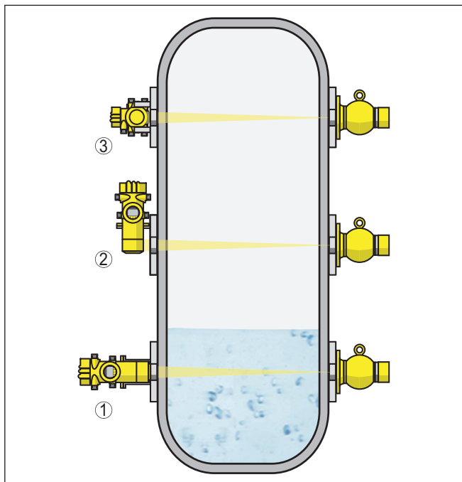
Fig. 5: Position de montage - Détection de niveau
