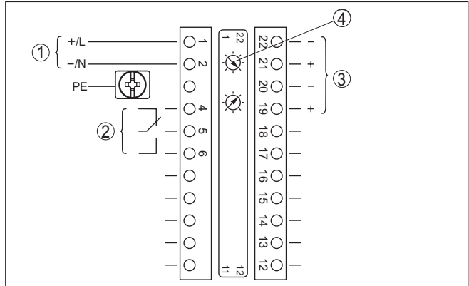
Fig. 14: Compartiment électronique et de raccordement (Ex d) des appareils avec sortie courant à sécurité intrinsèque
