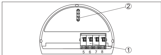
Fig. 13: Compartiment de réglage et de raccordement des appareils non Ex et appareils avec sortie courant non à sécurité intrinsèque
