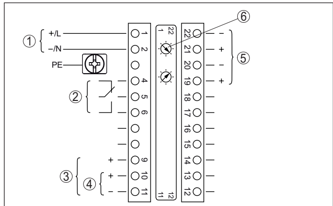
Fig. 12: Compartiment électronique et de raccordement des appareils non Ex et appareils avec sortie courant non à sécurité intrinsèque
