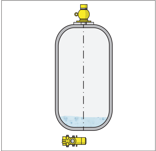
Fig. 6: Mesure de niveau - détection des quantités restantes sur une cuve de stockage
