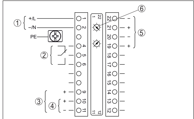
Fig. 8: Compartiment électronique et de raccordement des appareils non Ex et appareils avec sortie courant non à sécurité intrinsèque
