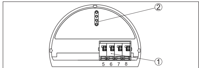
Fig. 9: Compartiment de réglage et de raccordement des appareils non Ex et appareils avec sortie courant non à sécurité intrinsèque
