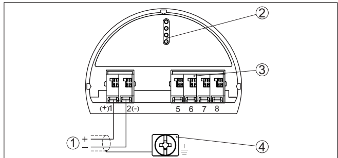
Fig. 15: Compartiment de réglage et de raccordement (Ex ia) des appareils avec sortie courant à sécurité intrinsèque
