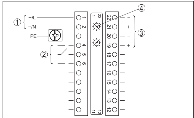
Fig. 10: Compartiment électronique et de raccordement (Ex d) des appareils avec sortie courant à sécurité intrinsèque
