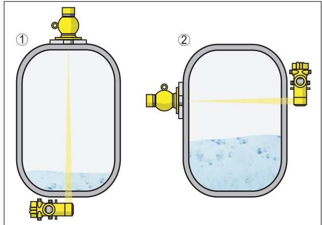
Fig. 3: MINITRAC 31 - Possibilités d'application
