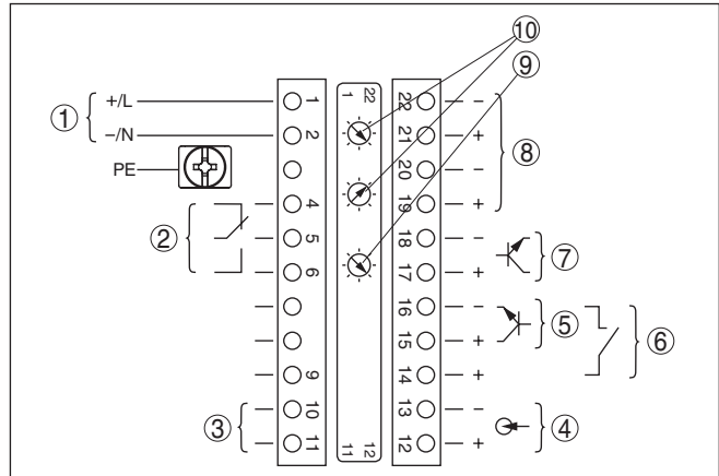
Fig. 15: Compartimento do sistema eletrônico e de conexão - em aparelhos Não-Ex e aparelhos com saída de sinal sem segurança intrínseca.
