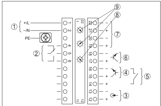
Fig. 17: Compartimento do sistema eletrônico e de conexão (EX d) em aparelhos com saída de sinal com segurança intrínseca
