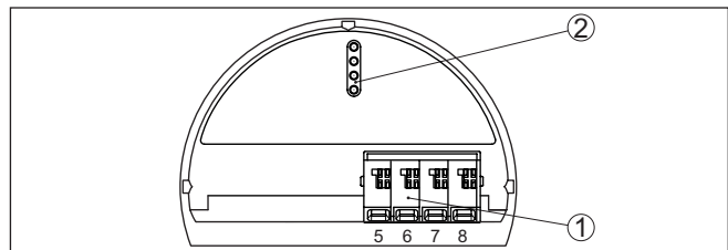
Fig. 16: Compartimento de configuração e de conexão - em aparelhos Não-Ex e aparelhos com saída de sinal sem segurança intrínseca.
