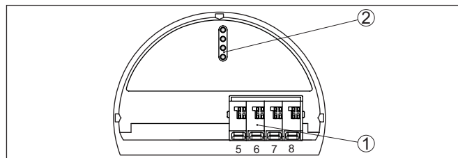
Fig. 16: Compartimiento de configuración y de conexión con equipos no Ex y equipos con salida de corriente sin seguridad intrínseca
