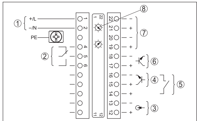
Fig. 17: Compartimiento del sistema electrónico y de conexión (Ex d) para equipos con salida de corriente con seguridad intrínseca
