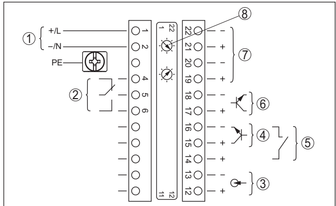
Fig. 13: Compartimento del sistema electrónico y de conexión (Ex d) para equipos con salida de corriente con seguridad intrínseca
