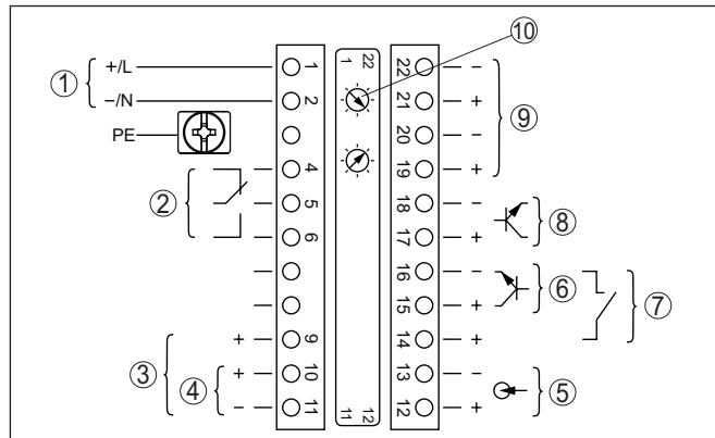
Fig. 15: Compartimiento del sistema electrónico y de conexiones para equipos no Ex y equipos con salida de corriente sin seguridad intrínseca
