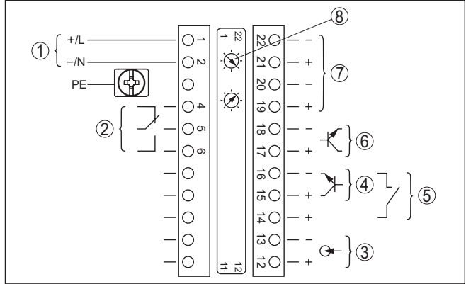
Res. 17: Bünyesinde güvenliği olan akım çıkışlı cihazlarda elektronik bölme ve bağlantı bölmesi (Ex d)
