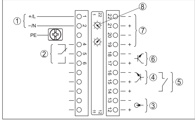
Res. 13: Bünyesinde güvenliği olan akım çıkışlı cihazlarda elektronik bölme ve bağlantı bölgesi (Ex d)
