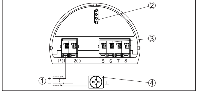
Res. 18: Bünyesinde güvenliği olan akım çıkışlı cihazlarda kumanda ve bağlantı bölümü (Ex ia)
