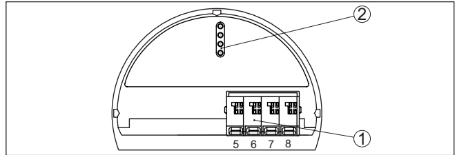
Res. 12: Ex olmayan cihazlar ve bünyesinde güvenliği olmayan akım çıkışlı cihazlarda kumanda ve bağlantı bölgesi
