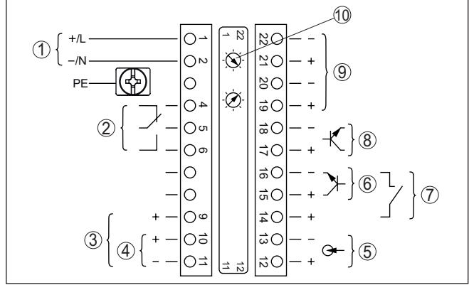
Res. 15: Ex olmayan cihazlar ve bünyesinde güvenliği olmayan akım çıkışlı cihazlarda elektronik bölme ve bağlantı bölgesi
