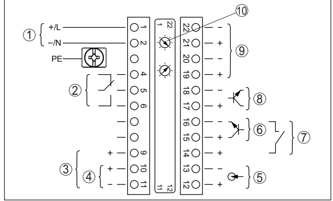
Res. 11: Ex olmayan cihazlar ve bünyesinde güvenliği olmayan akım çıkışlı cihazlarda elektronik bölme ve bağlantı bölgesi
