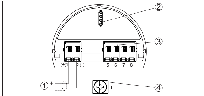
Res. 14: Bünyesinde güvenliği olan akım çıkışlı cihazlarda kumanda ve bağlantı bölgesi (Ex ia)
