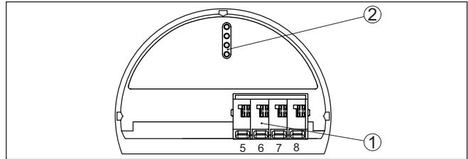
Res. 16: Ex olmayan cihazlar ve bünyesinde güvenliği olmayan akım çıkışlı cihazlarda kumanda ve bağlantı bölgesi
