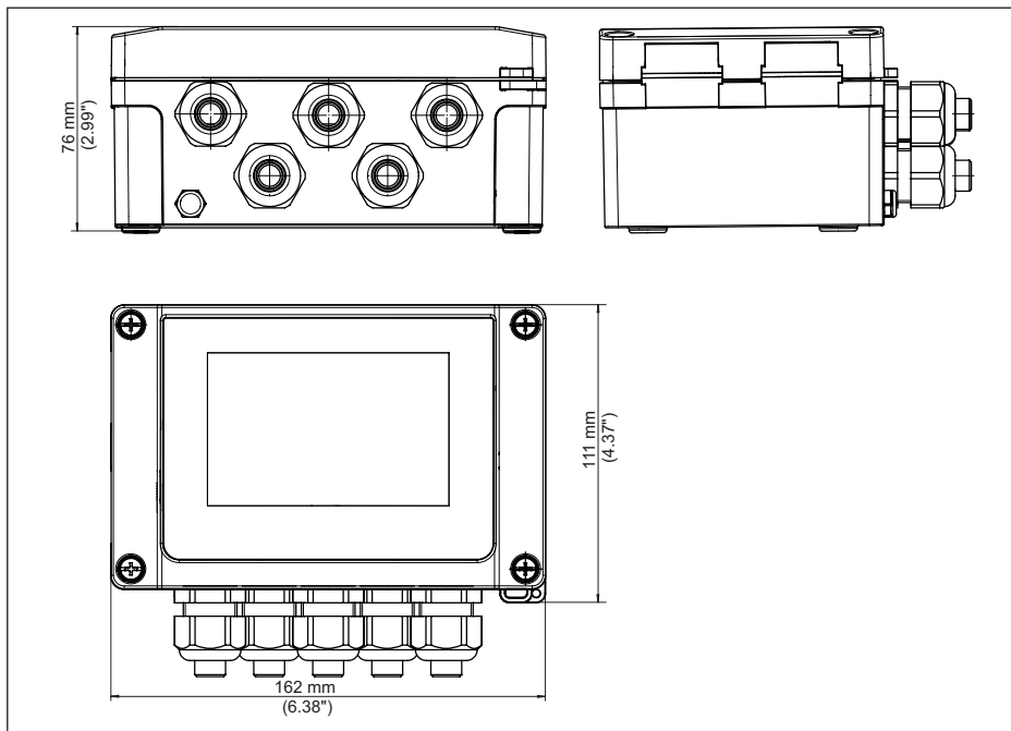
Fig. 22: Dimensões VEGAMET 841
