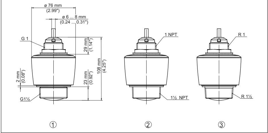
Res. 32: Ebatlar - VEGAPULS C 21
