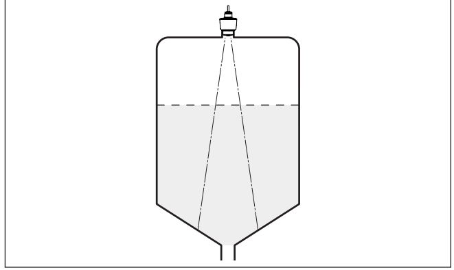
Res. 8: Radar sensörünün konik tabanlı haznelere montajı
