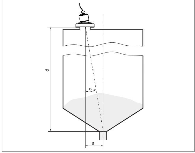
Res. 16: VEGAPULS C 21 hizalamaya göre kurulum için öneri
