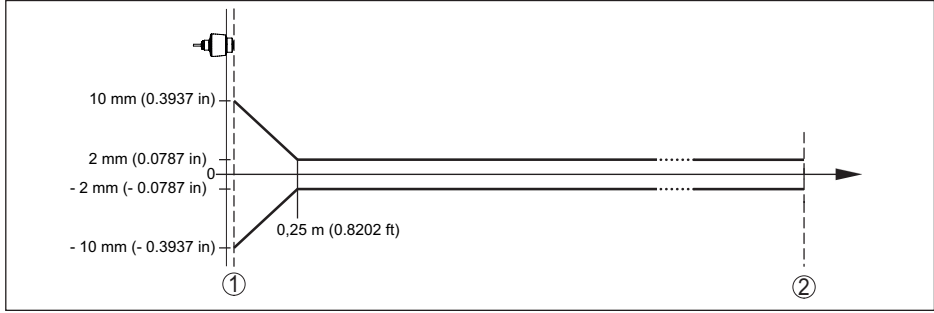
Res. 31: Referans koşullarına tabi ölçüm sapması 1)
