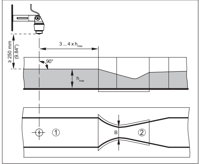
Res. 19: Khafagi venturi kanalı ile debi ölçümü: h_{maks.} = Kanalın maks. doldurulması; B = Kanalın en dar şekilde kapatılması
