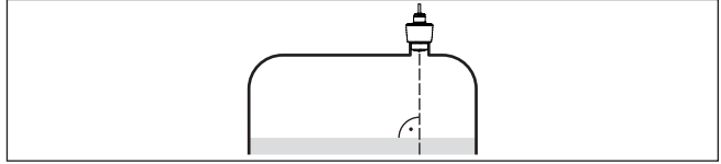
Res. 14: Sıvı içinde hizalama
