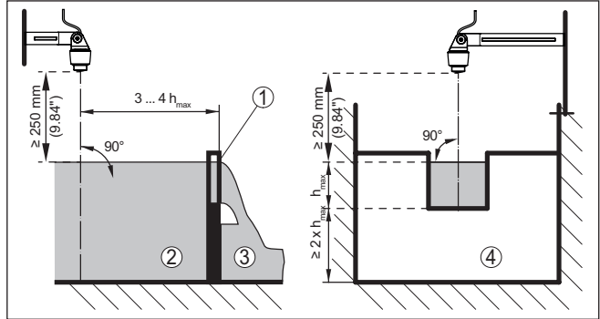
Res. 18: Dikdörtgen savaklı debi ölçümü: h_{\text{maks.}} = dikdörtgen savağın maks. dolumu
