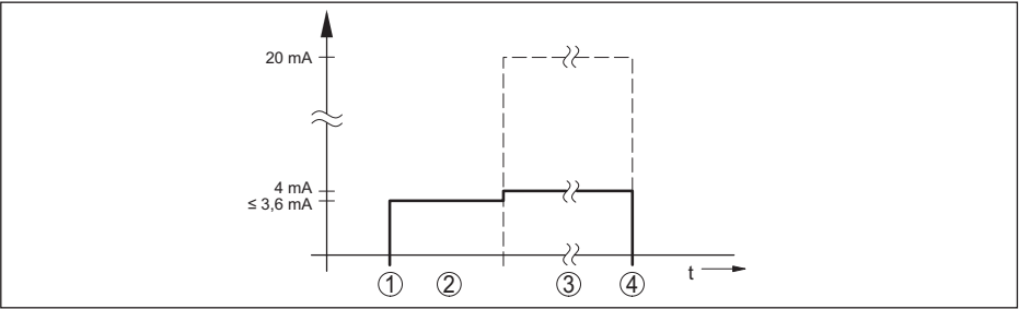
Res. 30: Başlatma süresi ve ölçüm değeri bildirisi
