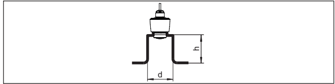
Res. 12: Boru soketleri ebatları standarttan farklı olduğunda
