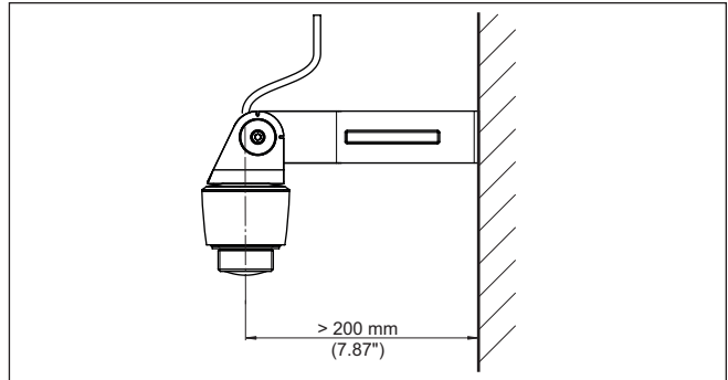
Res. 5: Bir montaj dirseği ile montaj
