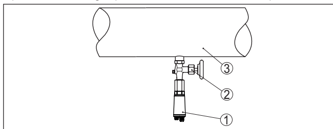
Figura 11: Configurazione di misura per la misura della pressione di processo di liquidi in tubazioni
