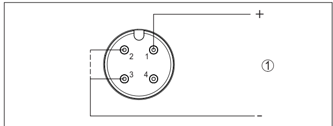
Figura 18: Schema di collegamento - bifilare 4 ... 20 mA - connettore M12 x 1
