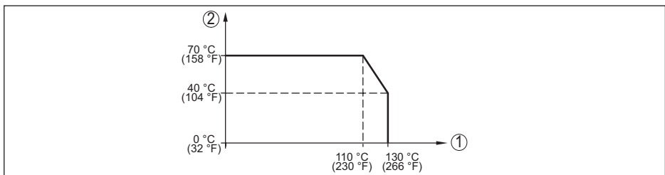
Figura 28: Derating di temperatura VEGABAR 29
