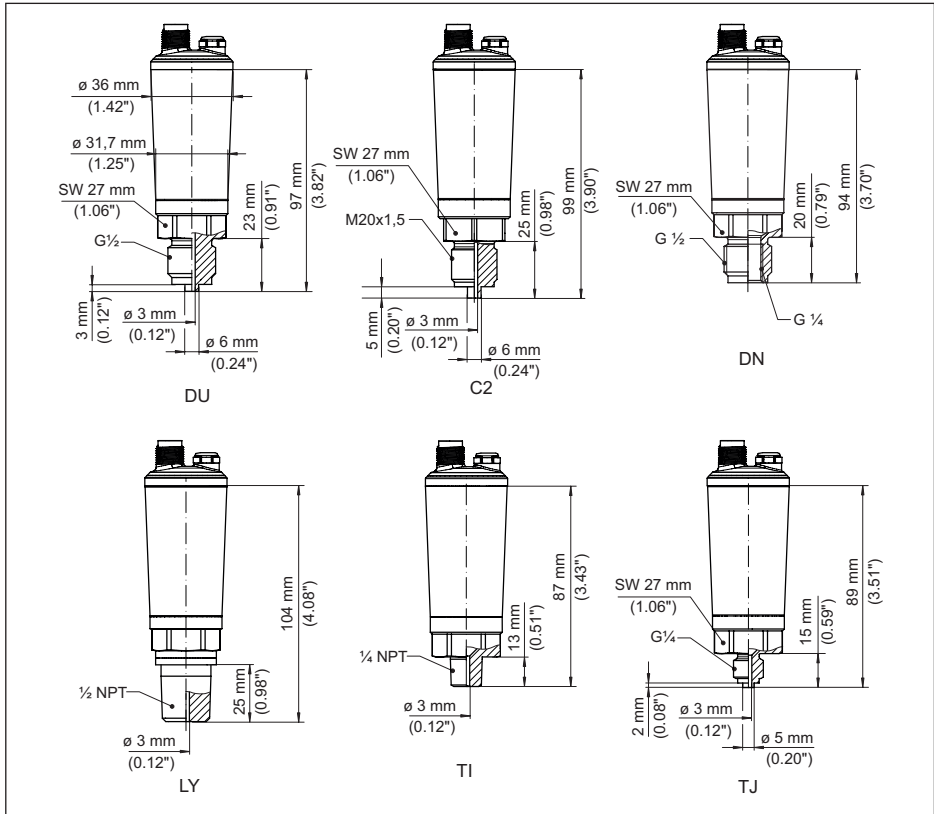
Figura 31: VEGABAR 29, attacco filettato non affacciato
