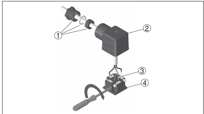
Figura 14: Collegamento ai morsetti a vite
