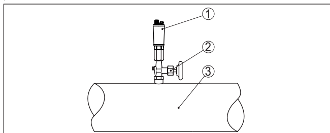
Figura 9: Configurazione di misura per la misura della pressione di processo di gas in tubazioni
