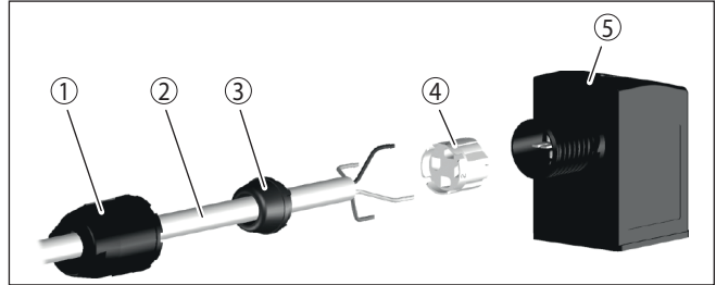
Figura 17: Collegamento del connettore a valvola ISO 4400 con tecnica di connessione con morsetti a perforazione di isolante
