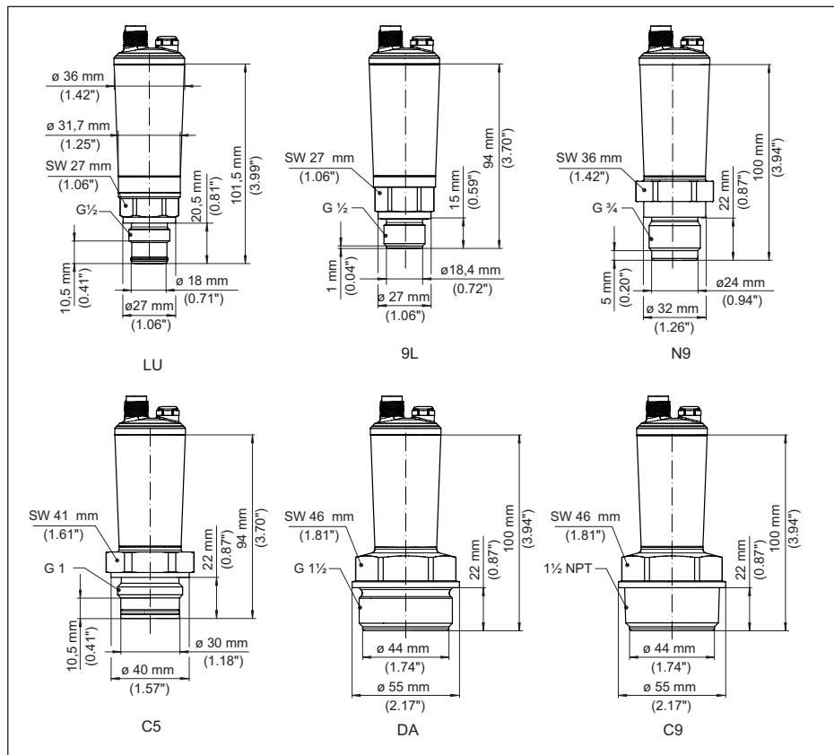
Figura 32: VEGABAR 29, attacco filettato affacciato
