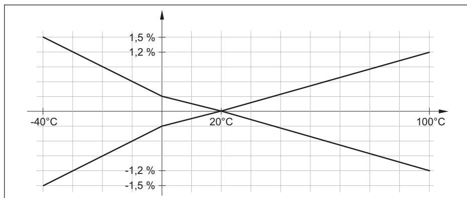
Figura 27: Errore di temperatura con TD 1 : 1
