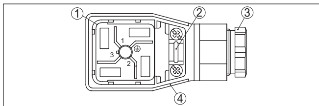
Figura 15: Rimozione dell'unità di connessione
