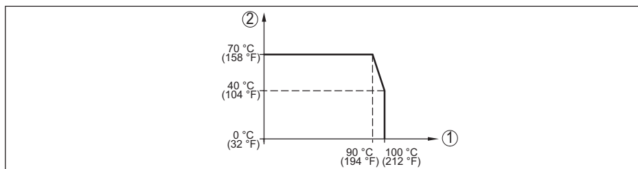
Figura 29: Derating termico VEGABAR 29, con comunicazione Bluetooth attivata
