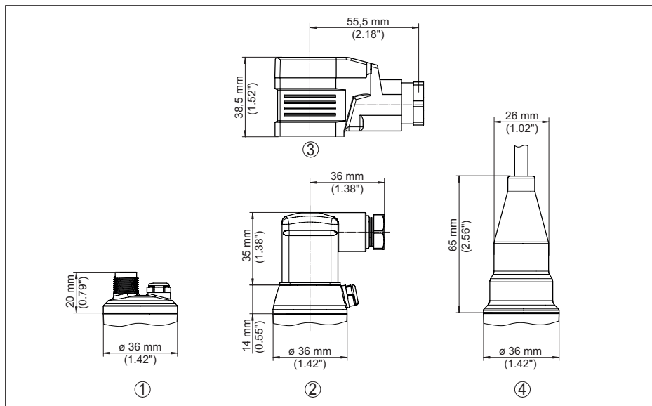
Figura 30: Tecnica di collegamento VEGABAR 29
