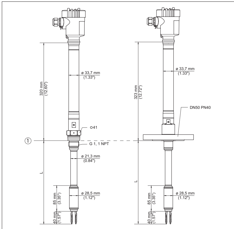
Fig. 22: VEGASWING 66, modelo para tubo
