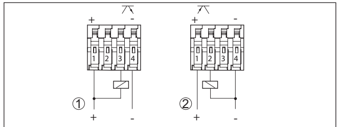
Fig. 12: Esquema de ligações
