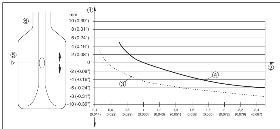
Figura 14: Influenza della densità del prodotto sul punto d'intervento
