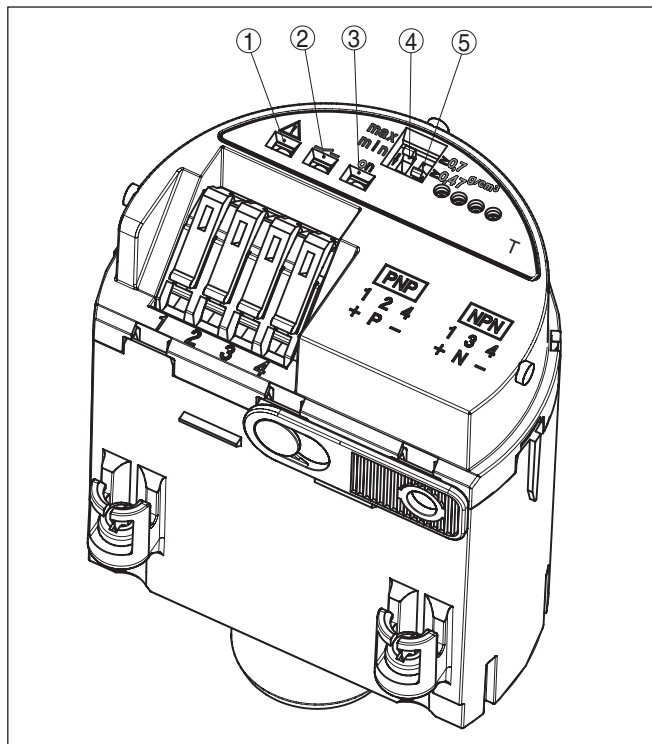
Figura 13: Unità elettronica - Uscita a transistor
