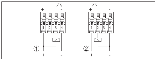
Figura 12: Schema di allacciamento
