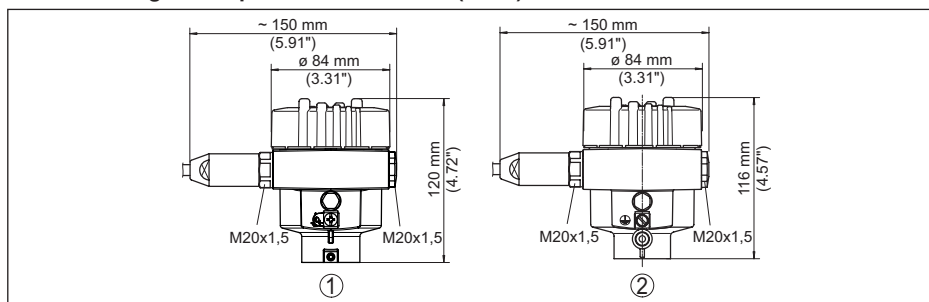
Figura 20: Le differenti custodie con grado di protezione IP66/IP68 (1 bar)
