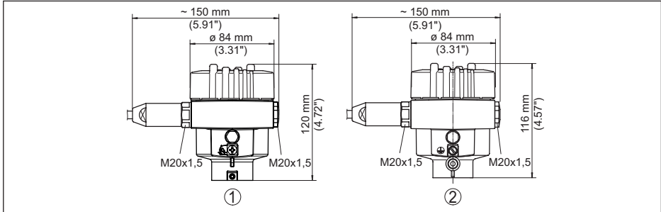
Res. 20: IP66/IP68 koruma tipinde gövde modelleri (1 bar)
