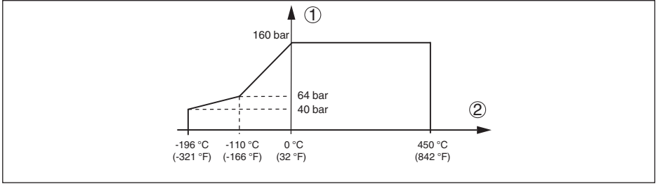
Res. 17: Proses sıcaklığı - Proses basıncı - 160 bar (2321 psig)'a kadar olan model
