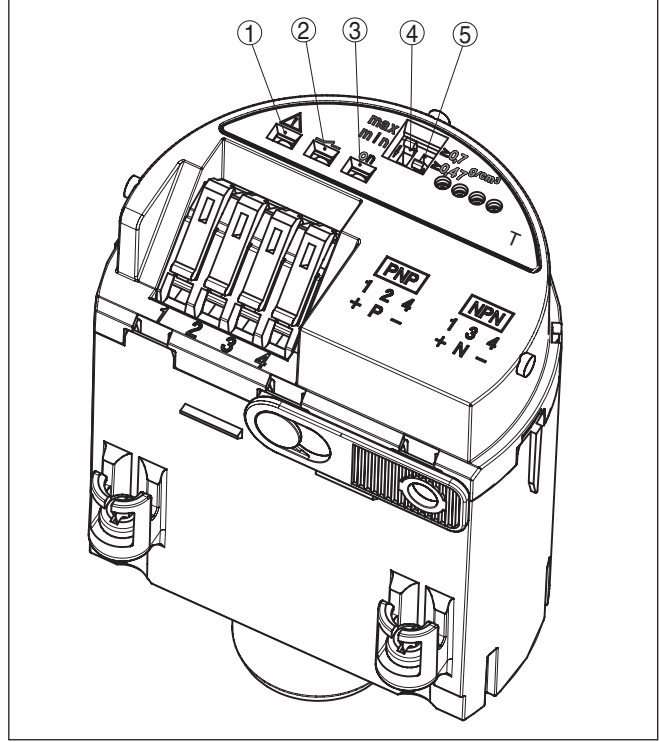
Res. 13: Elektronik modül - Transistör çıkışı
