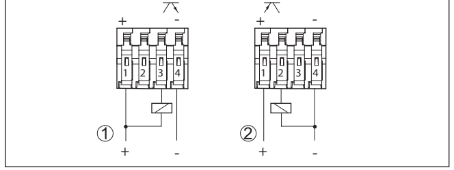
Res. 12: Bağlantı şeması
