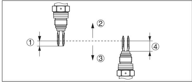
Fig. 3: Montagem vertical
