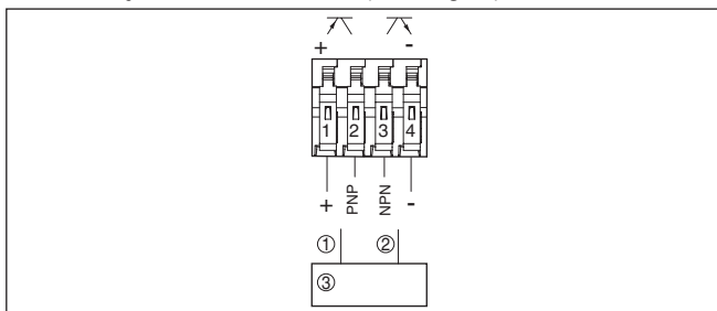
Fig. 13: Conexão para comandar um SPLC
