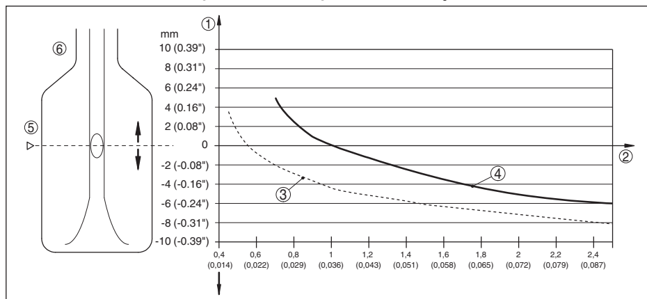
Fig. 15: Influência da densidade do produto sobre o ponto de comutação
