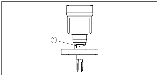
Fig. 6: Posição do garfo em modelos com flange
