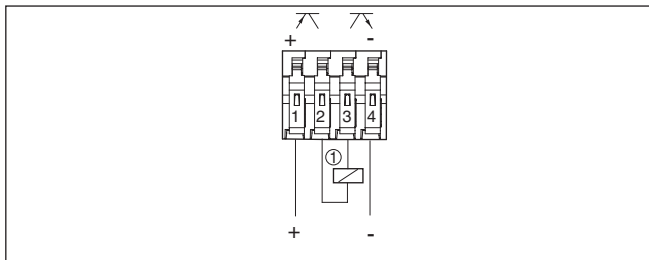
Fig. 12: Conexão para comandar, por exemplo, um relé 1 Carga
