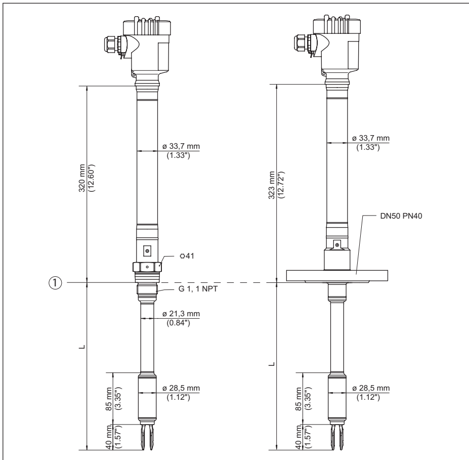
Fig. 21: VEGASWING 66, modelo para tubo
