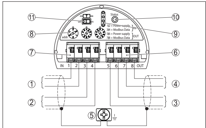
Fig. 4: Elektronicaruimte - aansluiting Daisy-Chain
