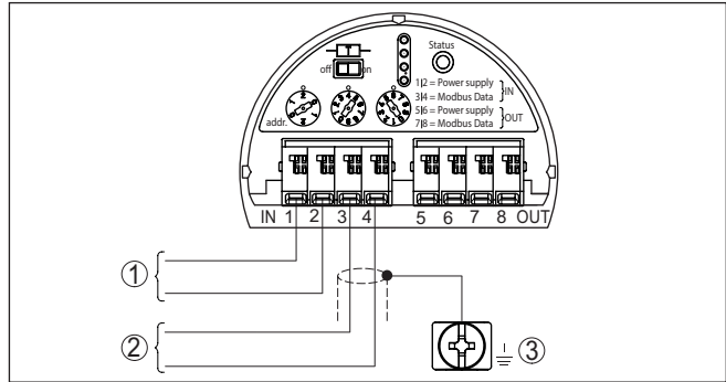
Fig. 5: Elektronica-ruimte - aansluiting met aftakkabel
