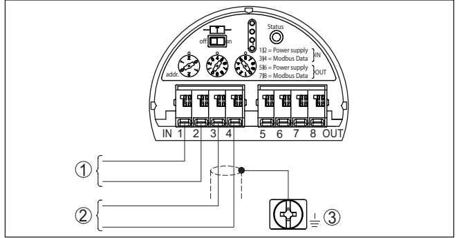
Res. 5: Elektronik bölme - Yan kablo ile bağlantı
