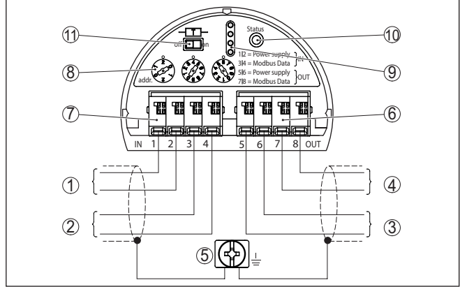
Res. 4: Elektronik bölme - Daisy-Chain bağlantısı
