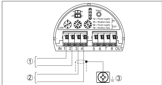
Abb. 5: Elektronikraum - Anschluss mit Stichleitung
