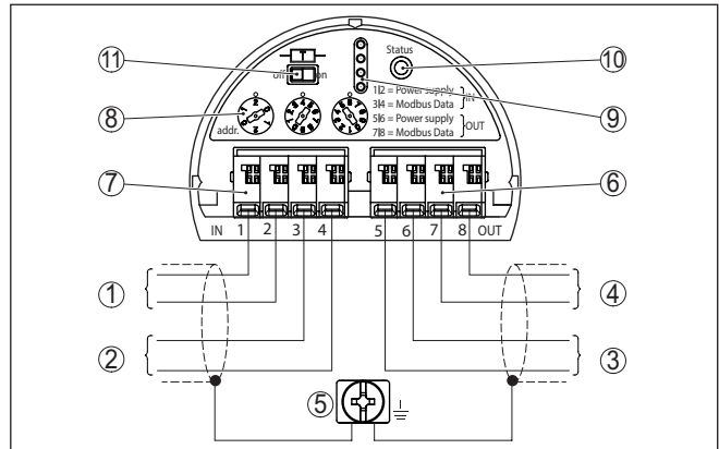
Abb. 4: Elektronikraum - Anschluss Daisy-Chain
