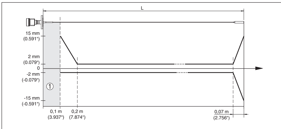
Fig. 29: Diferença de medição VEGAFLEX 83 em modelo com cabo de aço (revestido) com produto água
