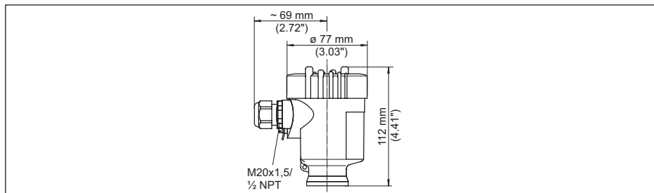
Fig. 32: Variantes da caixa com proteção IP66/IP67 (com o módulo de leitura e comando montado, a altura da caixa é aumentada em 9 mm/0,35 in)
