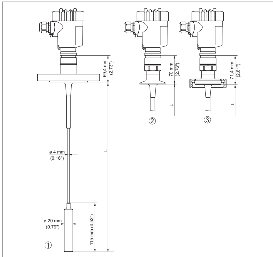
Fig. 37: VEGAFLEX 83, modelo com cabo de aço e peso tensor
