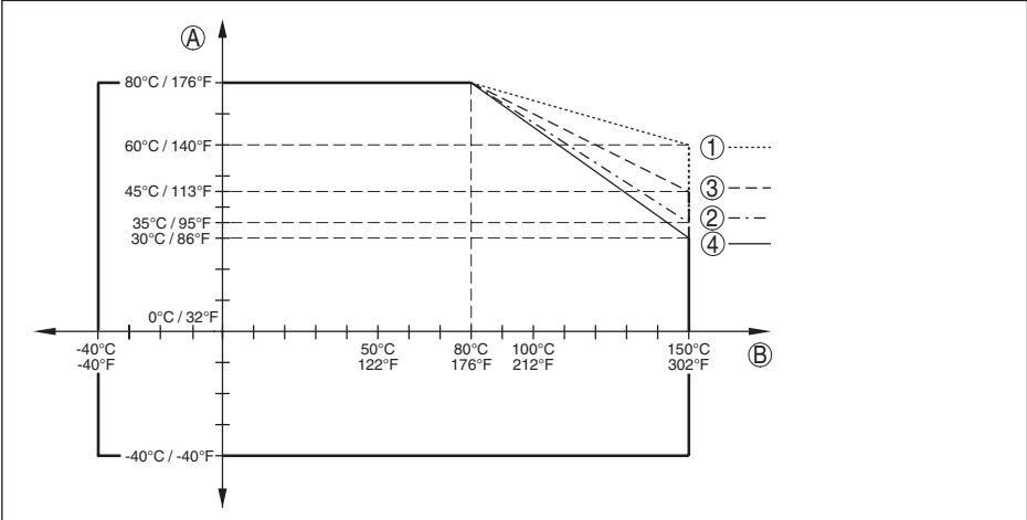
Fig. 31: Temperatura ambiente - Temperatura do processo, modelo padrão
