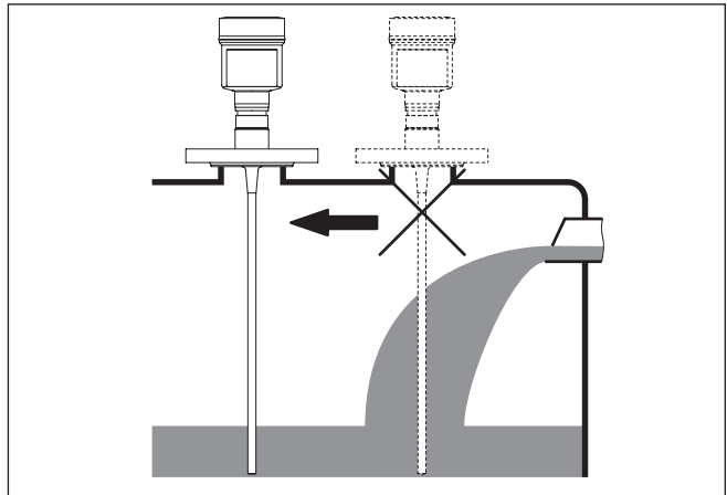
Fig. 8: Montagem do sensor no fluxo de entrada do produto
