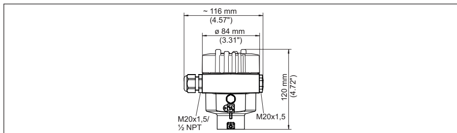
Fig. 33: Variantes da caixa com grau de proteção IP66/IP68 (0,2 bar), (com o módulo de visualização e configuração montado, a altura da caixa é aumentada em 9 mm/0,35 in)
