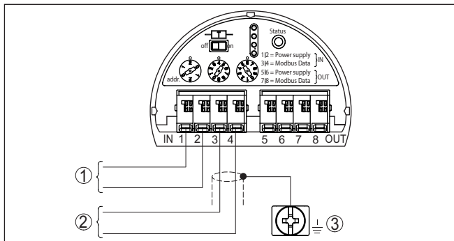
Fig. 12: compartimento do sistema eletrônico - Conexão com ramal
