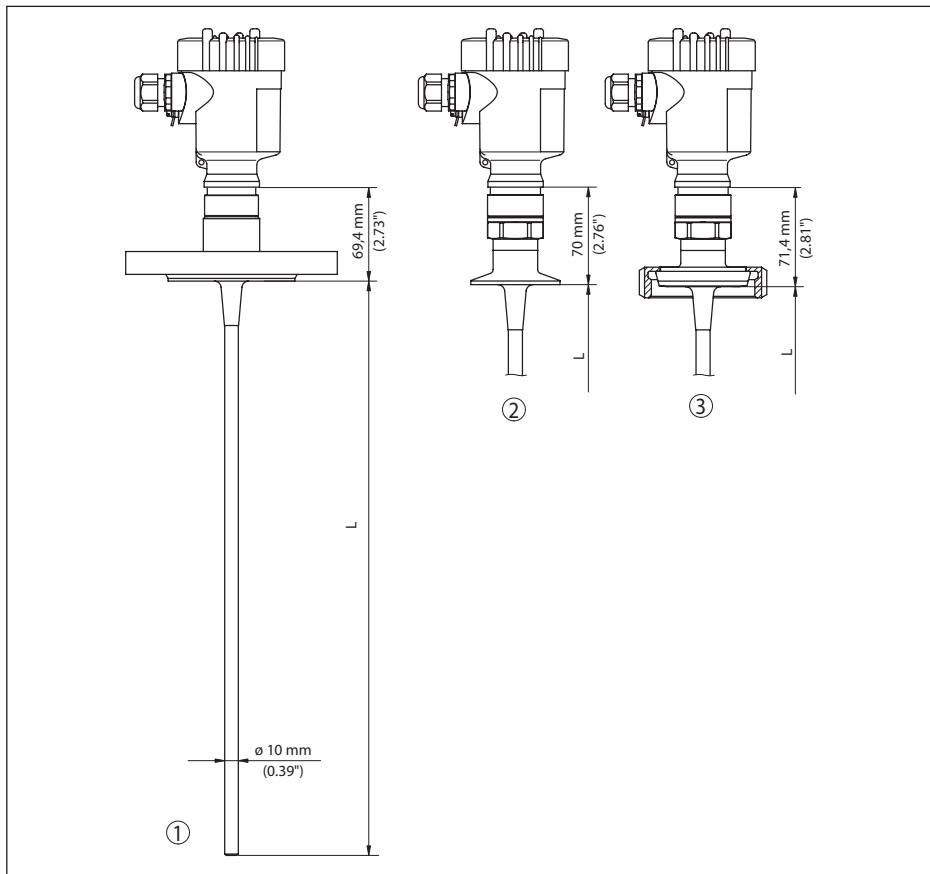
Fig. 38: VEGAFLEX 83, modelo com haste
