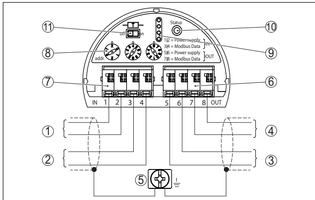
Fig. 11: Compartimento do sistema eletrônico - Conexão da Daisy-Chain
