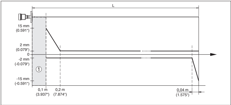
Fig. 27: Diferença de medição VEGAFLEX 83 em modelo com haste (revestida) com produto água
