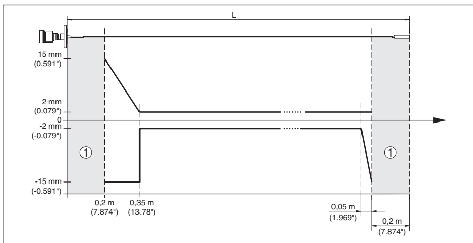
Fig. 30: Diferença de medição VEGAFLEX 83 em modelo com cabo (revestido) com produto óleo
