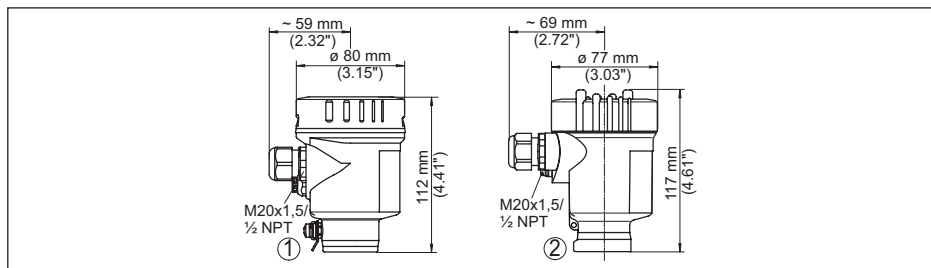
Fig. 35: Variantes da caixa com grau de proteção IP66/IP68 (0,2 bar), (com o módulo de visualização e configuração montado, a altura da caixa é aumentada em 9 mm/0,35 in)
