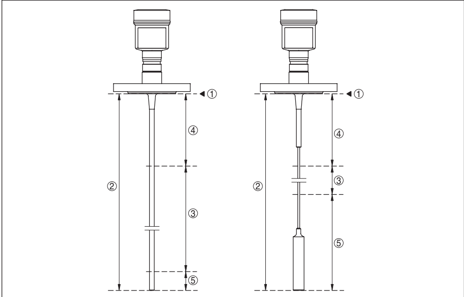
Fig. 26: Faixas de medição - VEGAFLEX 83
