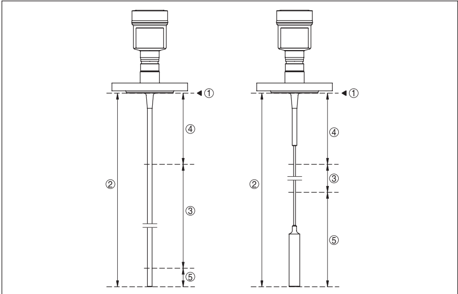
Fig. 26: Plages de mesure - VEGAFLEX 83
