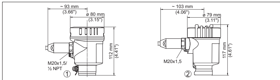
Fig. 36: Variantes de boîtier en protection IP66/IP68 (1 bar), (avec un module de réglage et d'affichage intégré, la hauteur du boîtier augmente de 9 mm/0.35 in)
