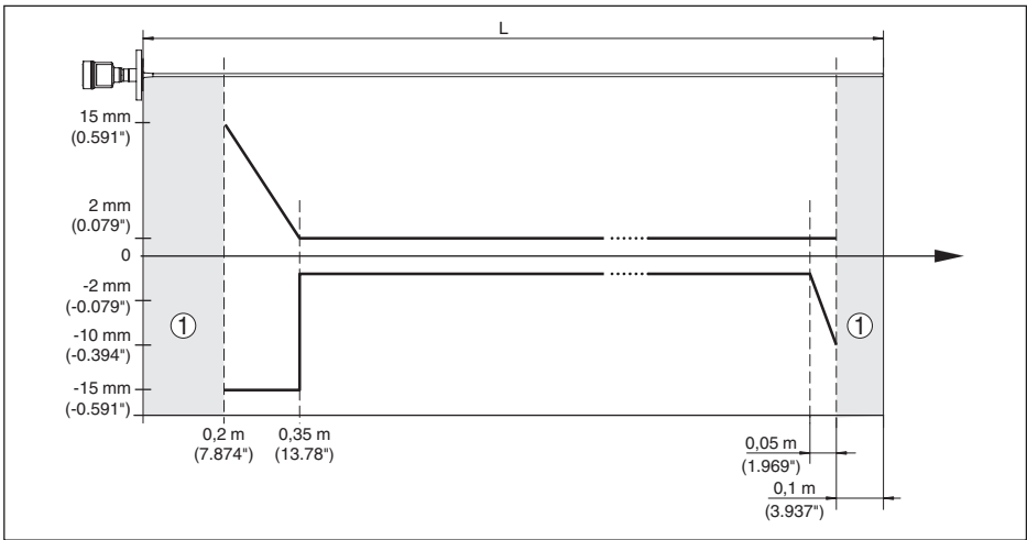
Fig. 28: Écart de mesure VEGAFLEX 83 en version tige (revêtue) dans l'huile
