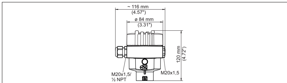
Fig. 33: Variantes de boîtier en protection IP66/IP68 (0,2 bar), (avec un module de réglage et d'affichage intégré, la hauteur du boîtier augmente de 9 mm/0.35 in)
