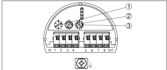
Fig. 13: Bouton de sélection d'adresse
