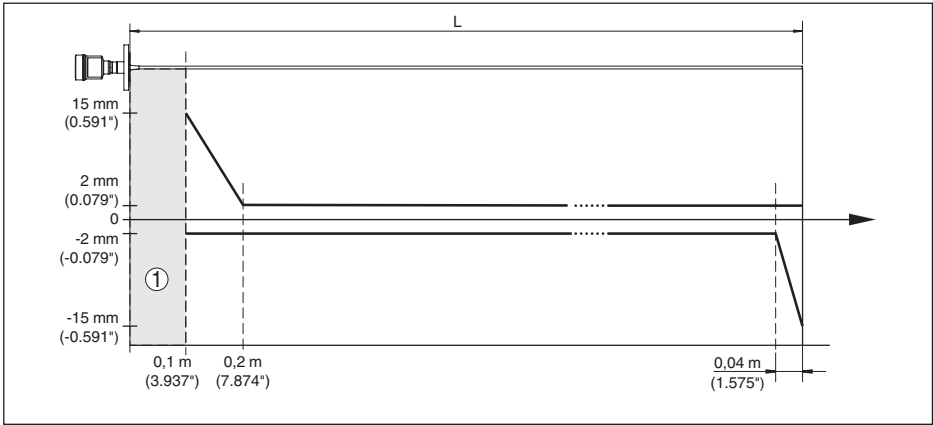
Fig. 27: Écart de mesure VEGAFLEX 83 en version tige (revêtue) dans l'eau
