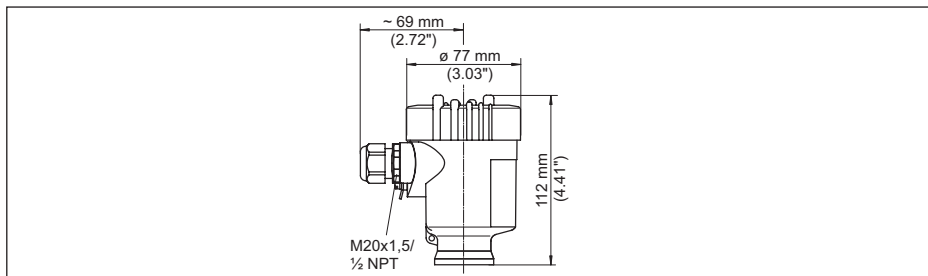
Fig. 32: Variantes de boîtier en protection IP66/IP67 (avec un module de réglage et d'affichage intégré, la hauteur du boîtier augmente de 9 mm/0.35 in)
