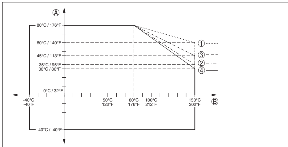
Fig. 31: Température ambiante - température process, version standard
