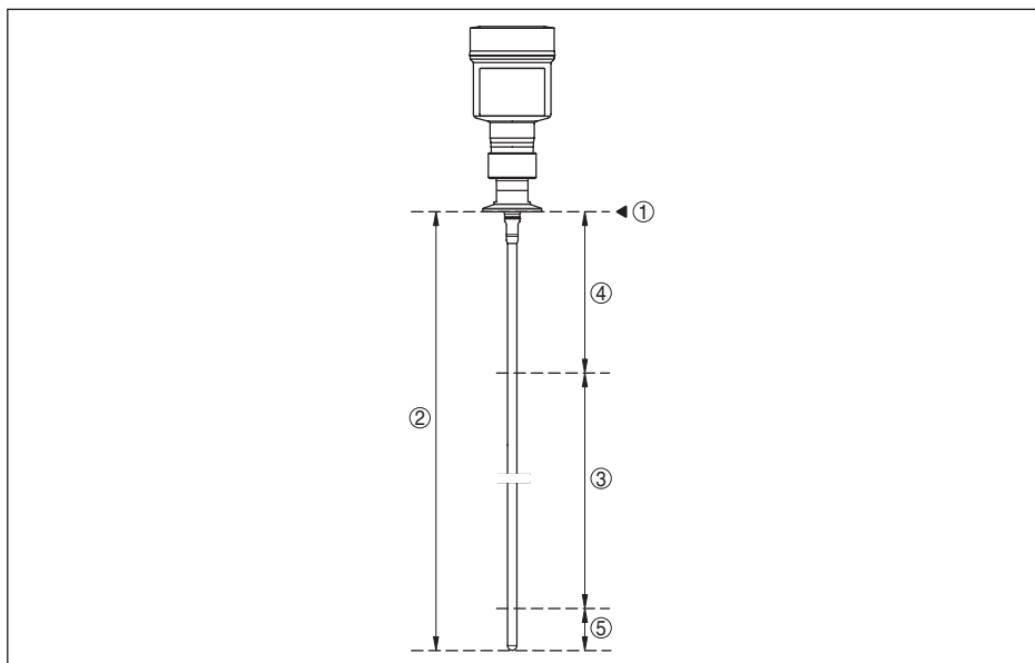
Rys. 29: Zakresy pomiarowe - VEGAFLEX 83
