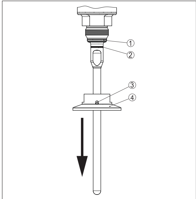
Rys. 28: Uszczelka przyłącza technologicznego
