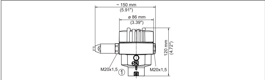
Rys. 35: Wersje wykonania obudowy ze stopniem ochrony IP66/IP68 (1 bar), (z zainstalowanym modulem wyświetlającym i obsługowym zwiększa się wysokość przyrządu o 9 mm/0.35 in)
