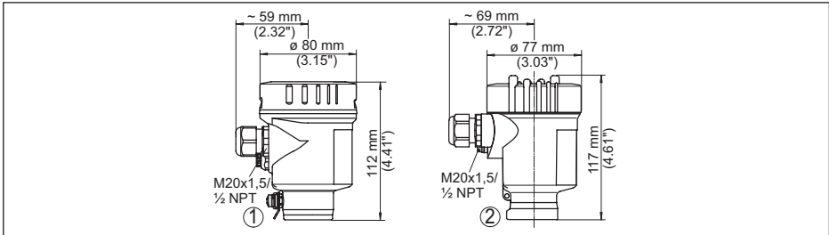
Rys. 36: Wersje wykonania obudowy ze stopniem ochrony IP66/IP68 (0,2 bar), (z zainstalowanym modulem wyświetlającym i obsługowym zwiększa się wysokość przyrządu o 9 mm/0.35 in)
