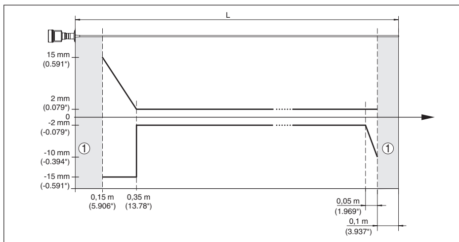
Rys. 31: Odchyłka pomiarowa VEGAFLEX 83 w wersji z falowodem prętowym w oleju jako medium
