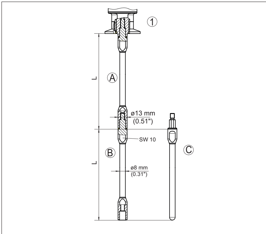
Rys. 40: Przedłużacze pręta \varnothing 8 \text{ mm} (0.315 in)
