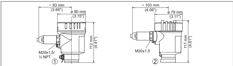
Rys. 37: Wersje wykonania obudowy ze stopniem ochrony IP66/IP68 (1 bar), (z zainstalowanym modulem wyświetlającym i obsługowym zwiększa się wysokość przyrządu o 9 mm/0.35 in)
