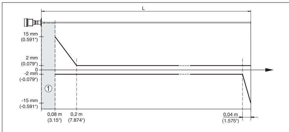
Rys. 30: Odchyłka pomiarowa VEGAFLEX 83 w wersji z falowodem prętowym w wodzie jako medium
