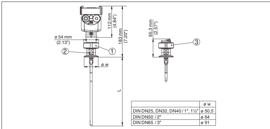
Rys. 39: VEGAFLEX 83, wersja z prętem \varnothing 8 mm (0.315 in), polerowany - wersja nadająca się do autoklawów
