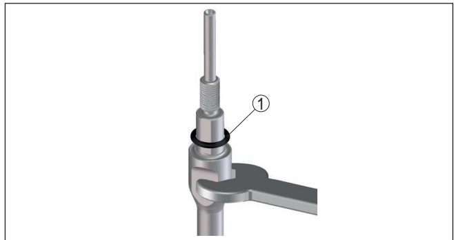
Rys. 26: Wymiana pręta falowodu
