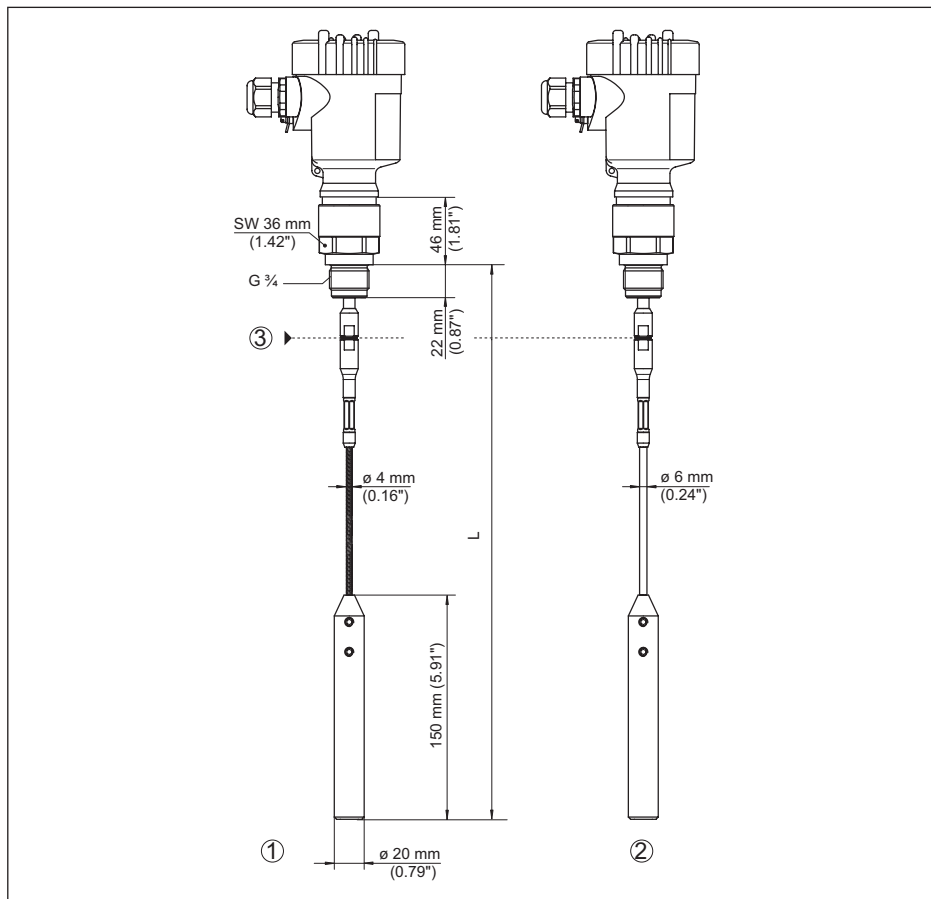
Fig. 41: VEGAFLEX 82, câble ø 4 mm (0.157 in), ø 6 mm (0.236 in) version fileté avec poids tenseur (tous les poids tenseurs avec filetage M12 pour anneau de levage)
