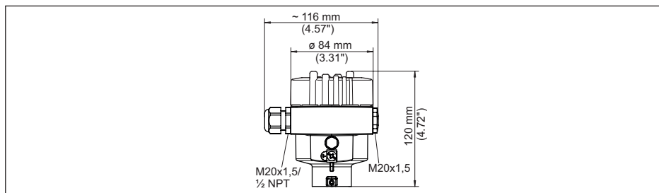
Fig. 37: Variantes de boîtier en protection IP66/IP68 (0,2 bar), (avec un module de réglage et d'affichage intégré, la hauteur du boîtier augmente de 9 mm/0.35 in)
