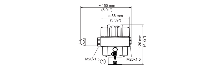
Fig. 38: Variantes de boîtier en protection IP66/IP68 (1 bar), (avec un module de réglage et d'affichage intégré, la hauteur du boîtier augmente de 9 mm/0.35 in)
