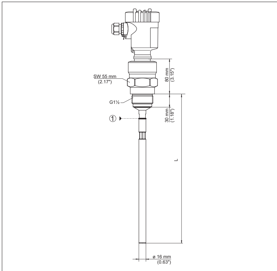
Fig. 43: VEGAFLEX 82, tige ø 16 mm (0.63 in), version filetée
