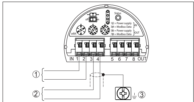
Fig. 11: Compartiment de l'électronique - Raccordement avec ramification
