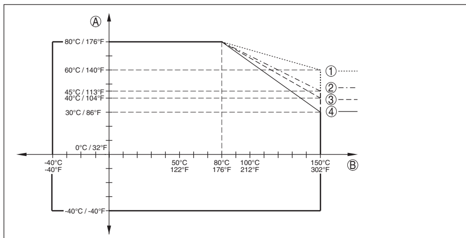
Fig. 34: Température ambiante - température process, version standard
