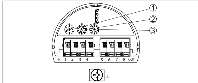
Fig. 12: Bouton de sélection d'adresse
