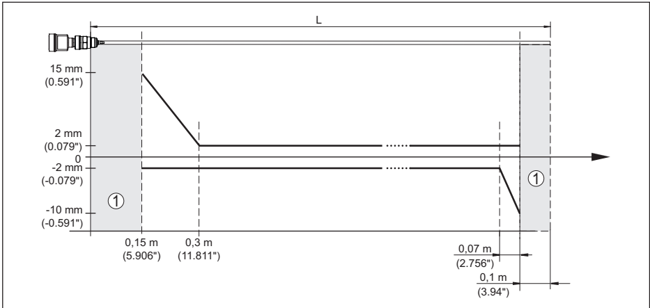
Fig. 32: Écart de mesure VEGAFLEX 82 en version tige
