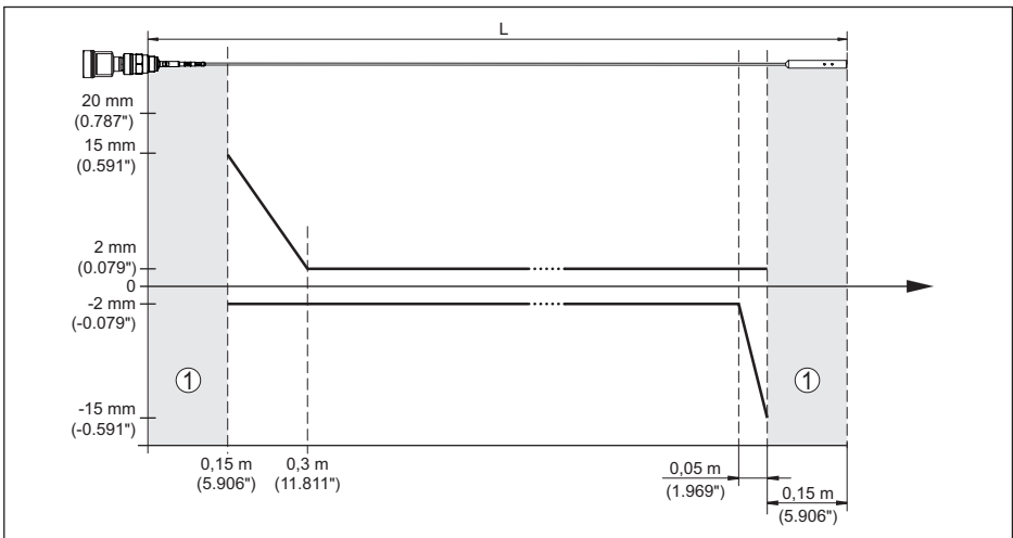
Fig. 33: Écart de mesure VEGAFLEX 82 en version câble
