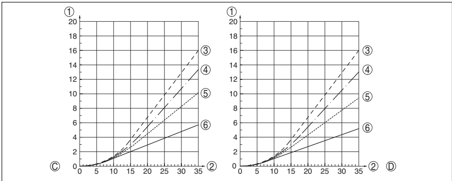
Fig. 28: Charge de traction max. avec sable et ciment - Câble : \phi 4 mm (0.157 in)
