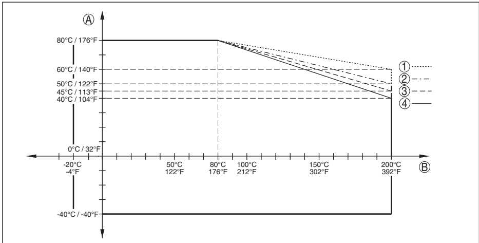
Fig. 35: Température ambiante - température process, version avec extension haute température
