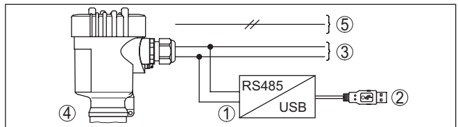
Fig. 20: Raccordement du PC à la ligne RS 485 via adaptateur d'interface
