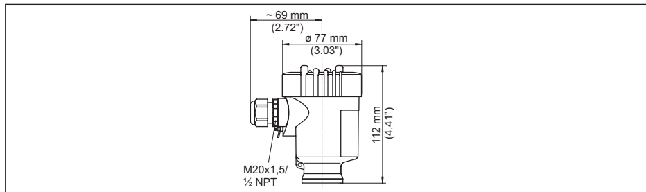
Fig. 36: Variantes de boîtier en protection IP66/IP67 (avec un module de réglage et d'affichage intégré, la hauteur du boîtier augmente de 9 mm/0.35 in)
