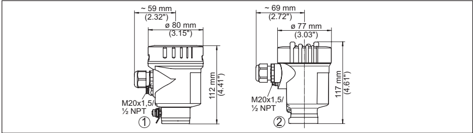
Fig. 39: Variantes de boîtier en protection IP66/IP68 (0,2 bar), (avec un module de réglage et d'affichage intégré, la hauteur du boîtier augmente de 9 mm/0.35 in)
