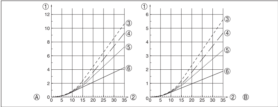
Fig. 27: Charge de traction max. avec céréales et granulés synthétiques - Câble : \phi 4 mm (0.157 in)
