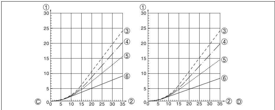
Fig. 30: Charge de traction max. avec sable et ciment - Câble : \varnothing 6 mm, \varnothing 11 mm, revêtu PA
