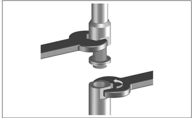
Fig. 25: Changer le câble de mesure ou la tige de mesure
