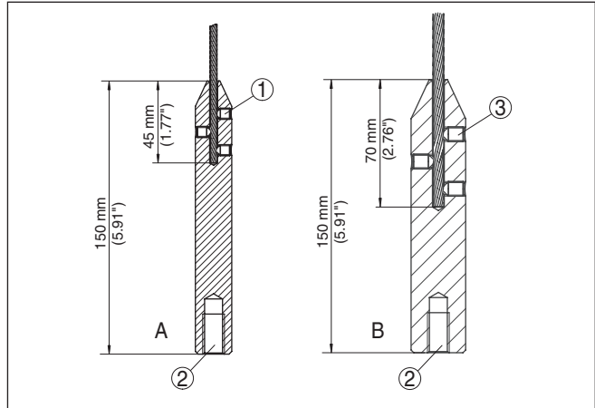
Fig. 26: Raccourcir le câble de la sonde
