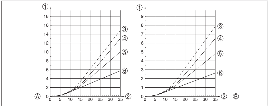
Fig. 29: Charge de traction max. avec céréales et granulés synthétiques - Câble : \varnothing 6 mm, \varnothing 11 mm, revêtu PA
