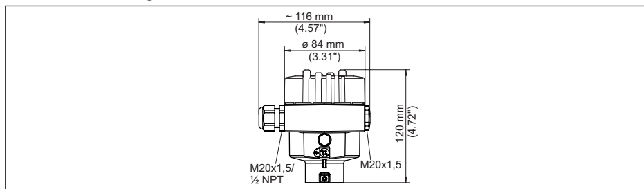
Fig. 28: Huisuitvoeringen in beschermingsklasse IP66/IP68 (0,2 bar), (met ingebouwde display- en bedieningsmodule wordt het huis 9 mm/0.35 in hoger)
