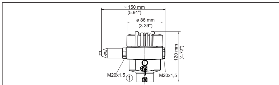
Fig. 29: Huisuitvoeringen in beschermingsklasse IP66/IP68 (1 bar), (met ingebouwde display- en bedieningsmodule wordt het huis 9 mm/0.35 in hoger)
