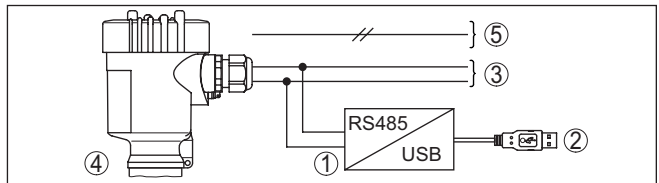
Fig. 17: Aansluiting van de PC via interface-adapter op de RS 485-kabel
