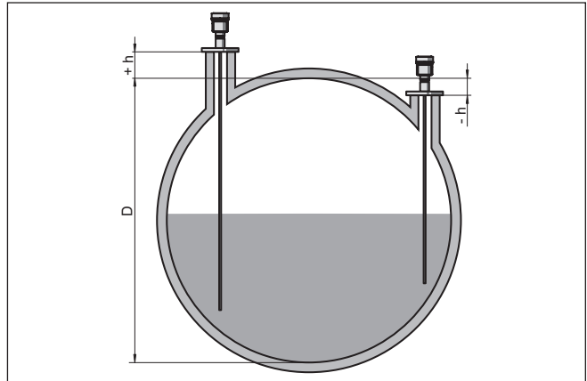
Fig. 13: Tankhoogte en sokcorrectiewaarde
