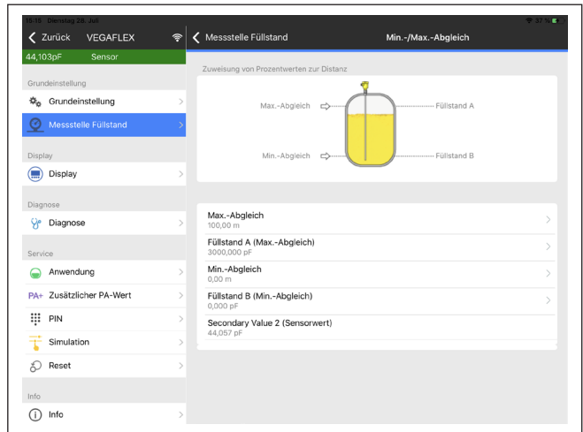
Fig. 15: Voorbeeld van een app-aanzicht - inbedrijfname sensorinregeling
