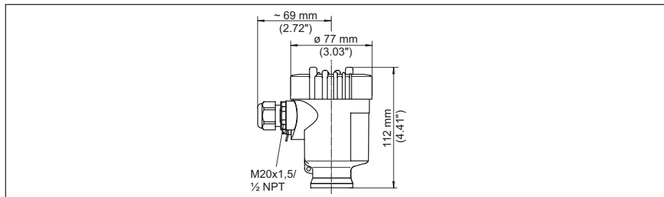
Fig. 27: Huisuitvoeringen in beschermingsklasse IP66/IP67 (met ingebouwde aanwijs- en bedieningsmodule wordt het huis 9 mm hoger)
