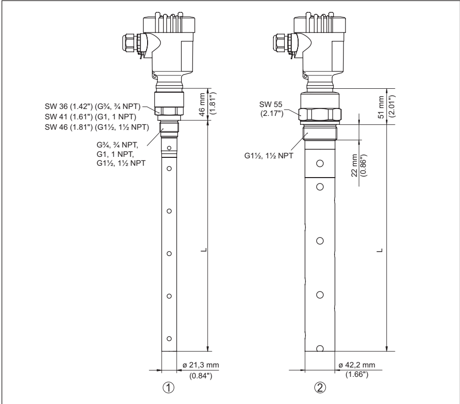
Fig. 32: VEGAFLEX 81, schroefdraaduitvoering
