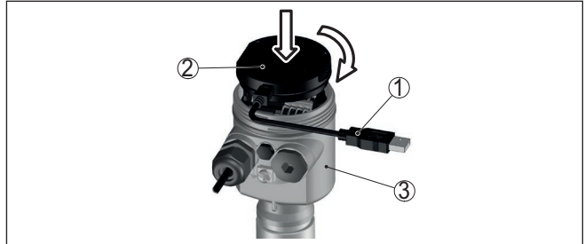
Fig. 16: Aansluiting van de PC via interface-adapter direct op de sensor
