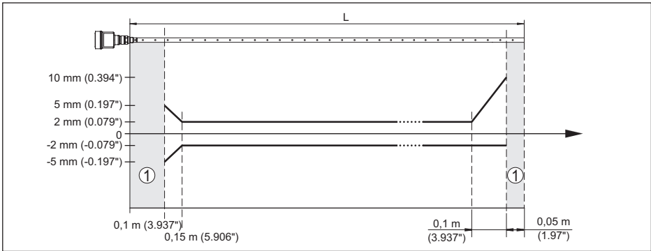
Fig. 24: Meets Nauwkeurigheid VEGAFLEX 81 in coaxuitvoering in medium olie
