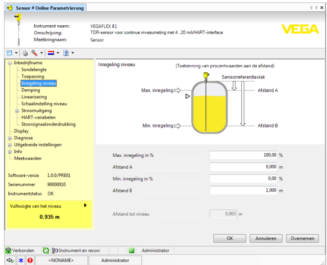
Fig. 18: Voorbeeld van een DTM-aanzicht
