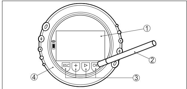
Fig. 12: Display- en bedieningselement - met bediening via magneetpen
