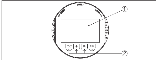
Fig. 11: Aanwijs- en bedieningselementen
