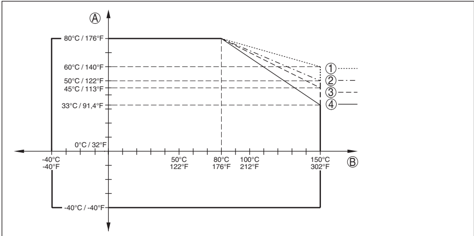
Fig. 25: Omgevingstemperatuur - procestemperatuur standaarduitvoering
