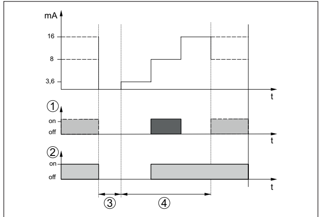
Abb. 4: Ablaufdiagramm eines korrekten Einschaltimpulses
