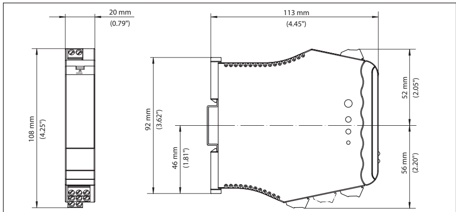
Abb. 6: Maße VEGATOR 121
