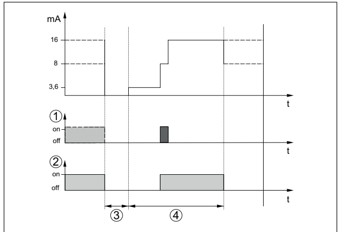
Abb. 5: Ablaufdiagramm eines falschen Einschaltimpulses
