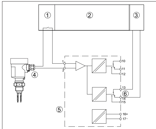
Abb. 3: Automatisierte Funktionsprüfung via Störmelderelais und SPS
