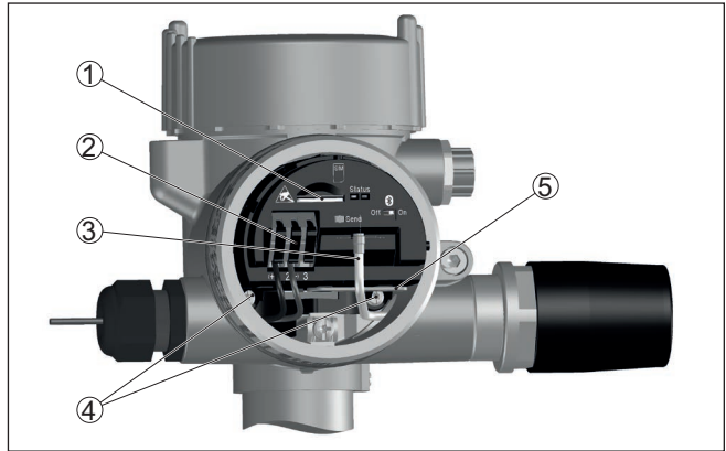
Abb. 1: Anschlussleitungen entfernen und Halteschrauben lösen
