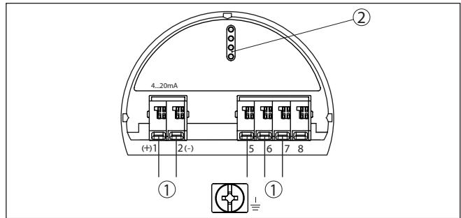
Rys. 3: Komora modułu elektronicznego - obudowa dwukomorowa
