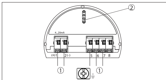
Fig. 3: Compartimento do sistema eletrônico - Caixa de duas câmaras
