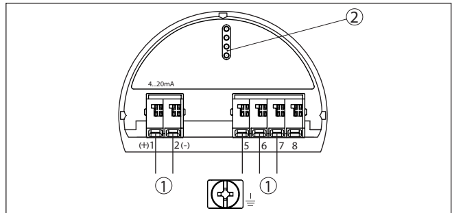
Fig. 3: Elektronicaruimte - tweekamerbehuizing
