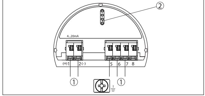
Res. 3: Elektronik bölümü - iki hücreli gövde
