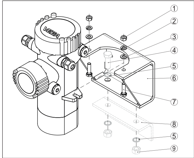
Fig. 3: Montagem do adaptador (modelo padrão)
