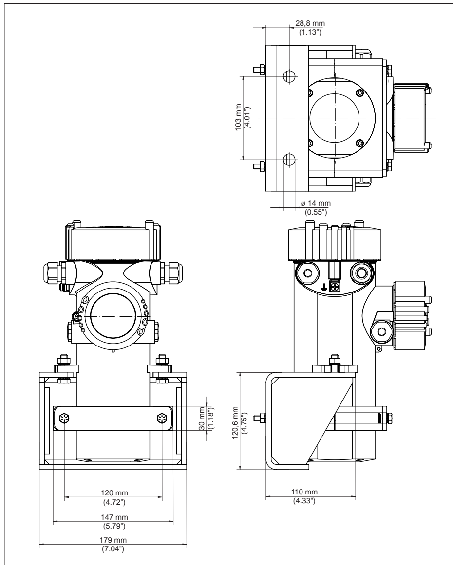
Fig. 6: Adaptador de montagem PTB 9, modelo à prova de vibrações
