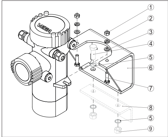
Figura 3: Montaggio dell'adattatore di montaggio (esecuzione standard)
