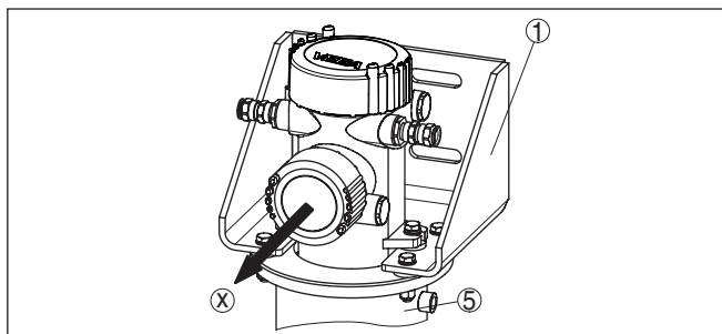
Fig. 3: Direção da montagem do sensor para o ângulo de fixação dos apoios
