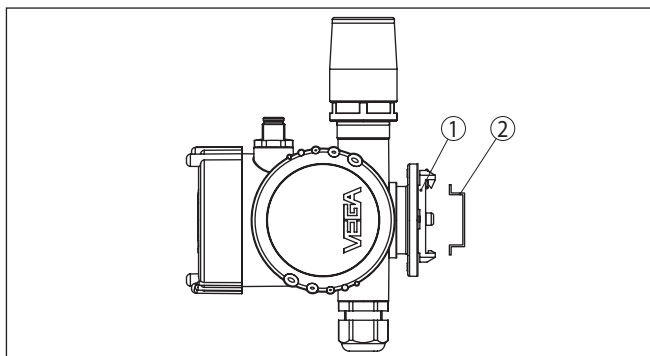
Fig. 3: PLICSMOBILE T81 para montagem em trilho
