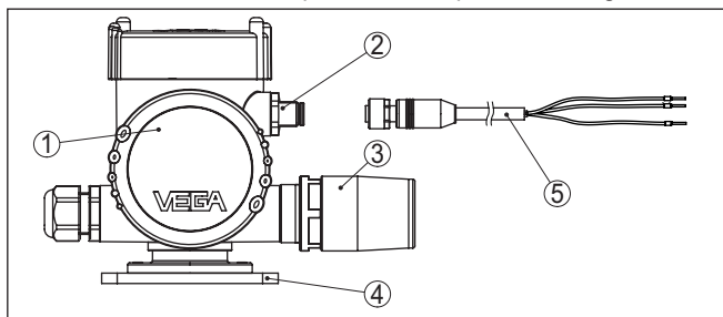
Fig. 1: PLICSMOBILE T81
