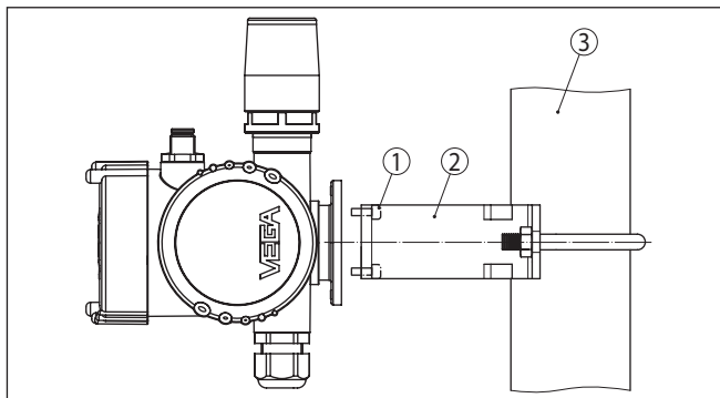
Fig. 4: PLICSMOBILE T81 para a montagem em tubo
