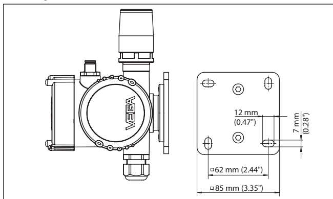
Fig. 2: PLICSMOBILE T81 para a montagem na parede. Placa de montagem vista de baixo.
