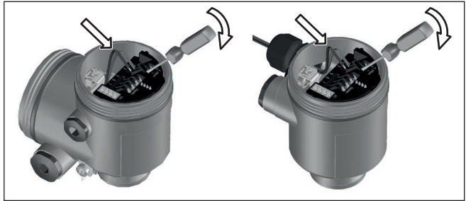
Abb. 3: Anschlusschritte 6 und 7
