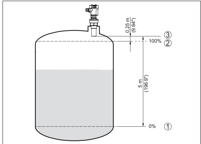
Fig. 7: Parametrevoorbeeld min.-/max.-inregeling
