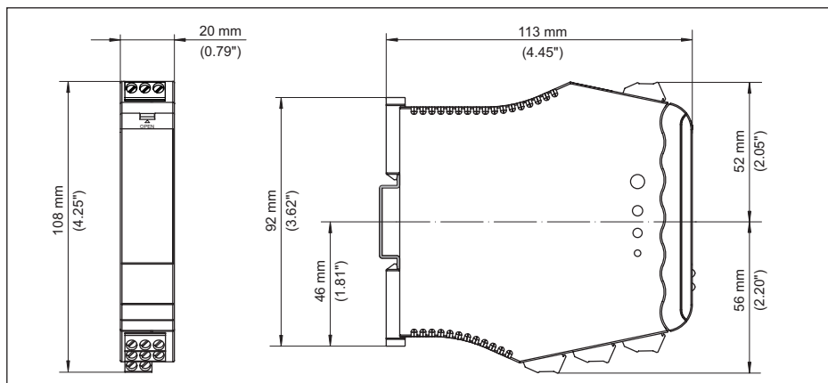
Figura 7: Dimensioni VEGATOR 131
