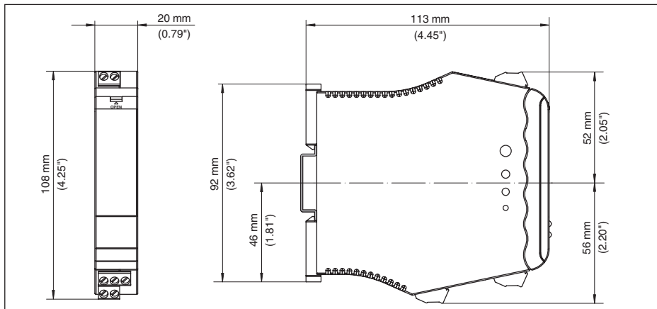
Fig. 2: Dimensões VEGATRENN 141
