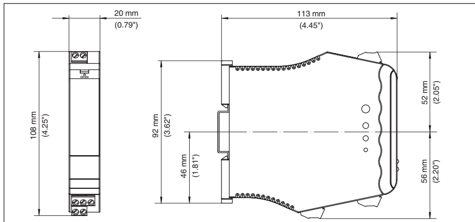
Figura 2: Dimensioni VEGATRENN 141
