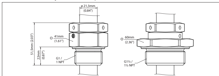
Fig. 2: União roscada de fixação ARV-SG63.4, tensão de operação: +0,1 bar (1.45 psig) para VEGASWING 63
