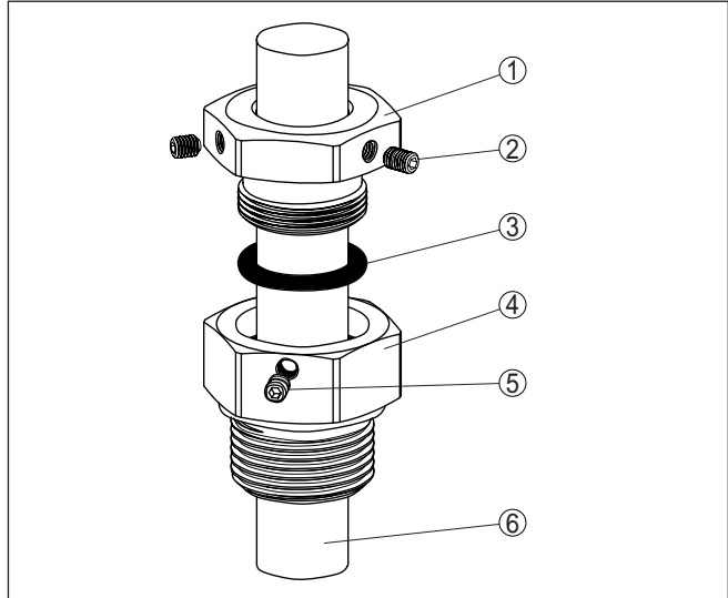
Fig. 1: União rosca de fixação ARV-SG63.4, +0,1 bar (1.45 psig)
