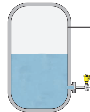
Livello: misura di livello con sistema di separazione applicato su un lato (CSS)
